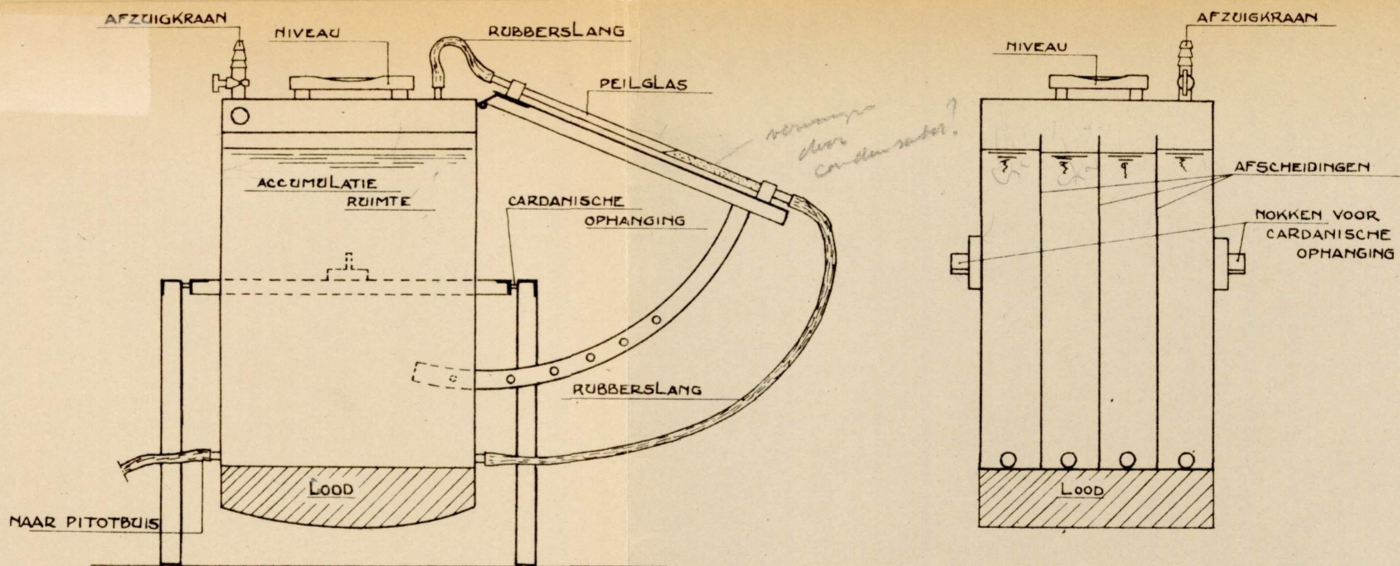
MANOMETERINRICHTING SCHAAL ± 1:5
