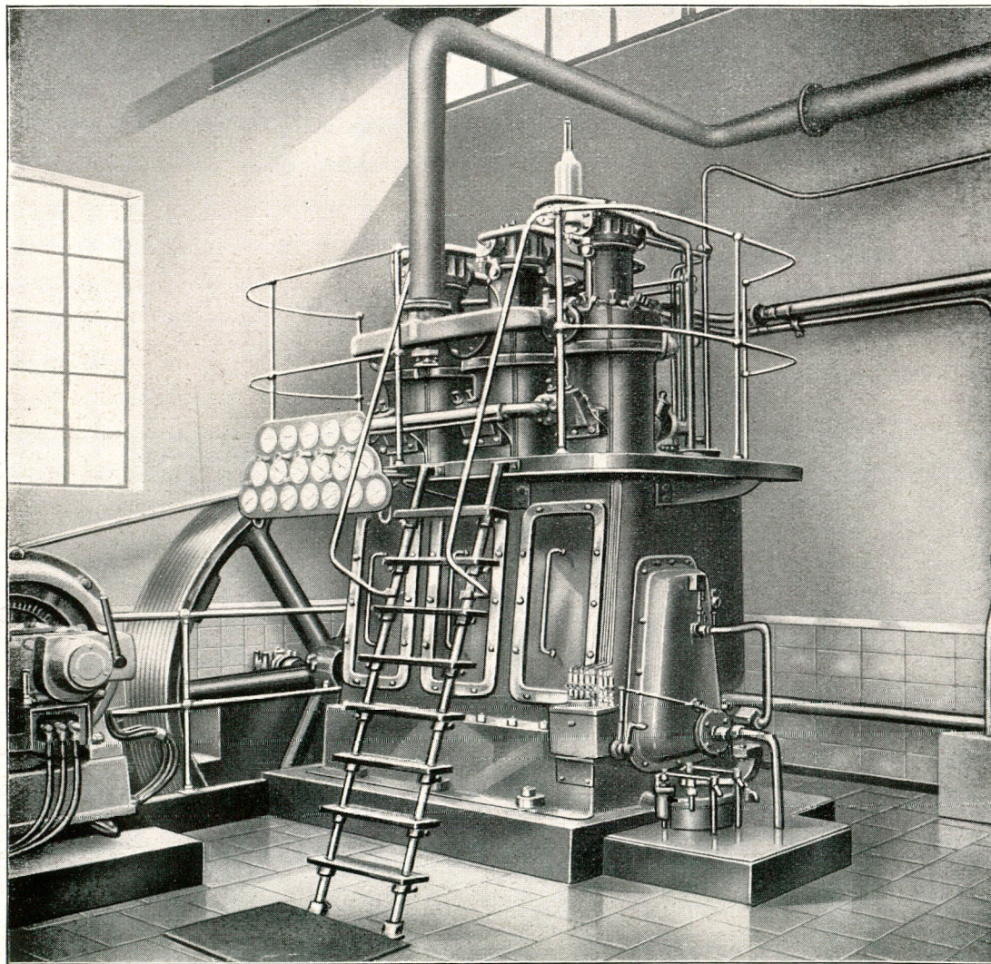
Vijftredige luchtcompressor, 500 M 3 /uur, 200 atm.
