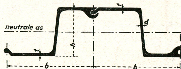
Bulbklauwen-Profiel
