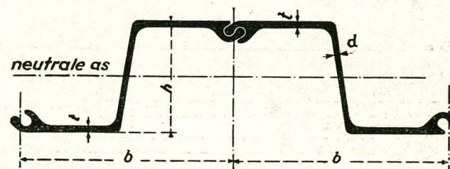
Dubbelklauwen-Profiel
