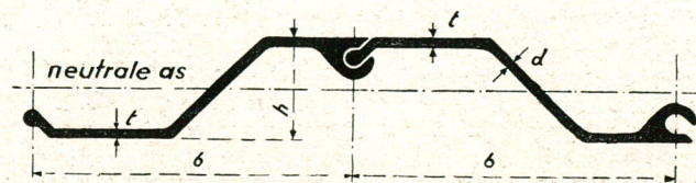
Speciaal-Profiel
