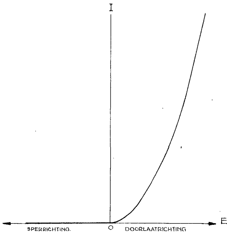
ALGEMENE STROOMSPANNINGS KARAKTERISTIEK VAN METAAL-GELUKRICHTERS. FIG 17.
