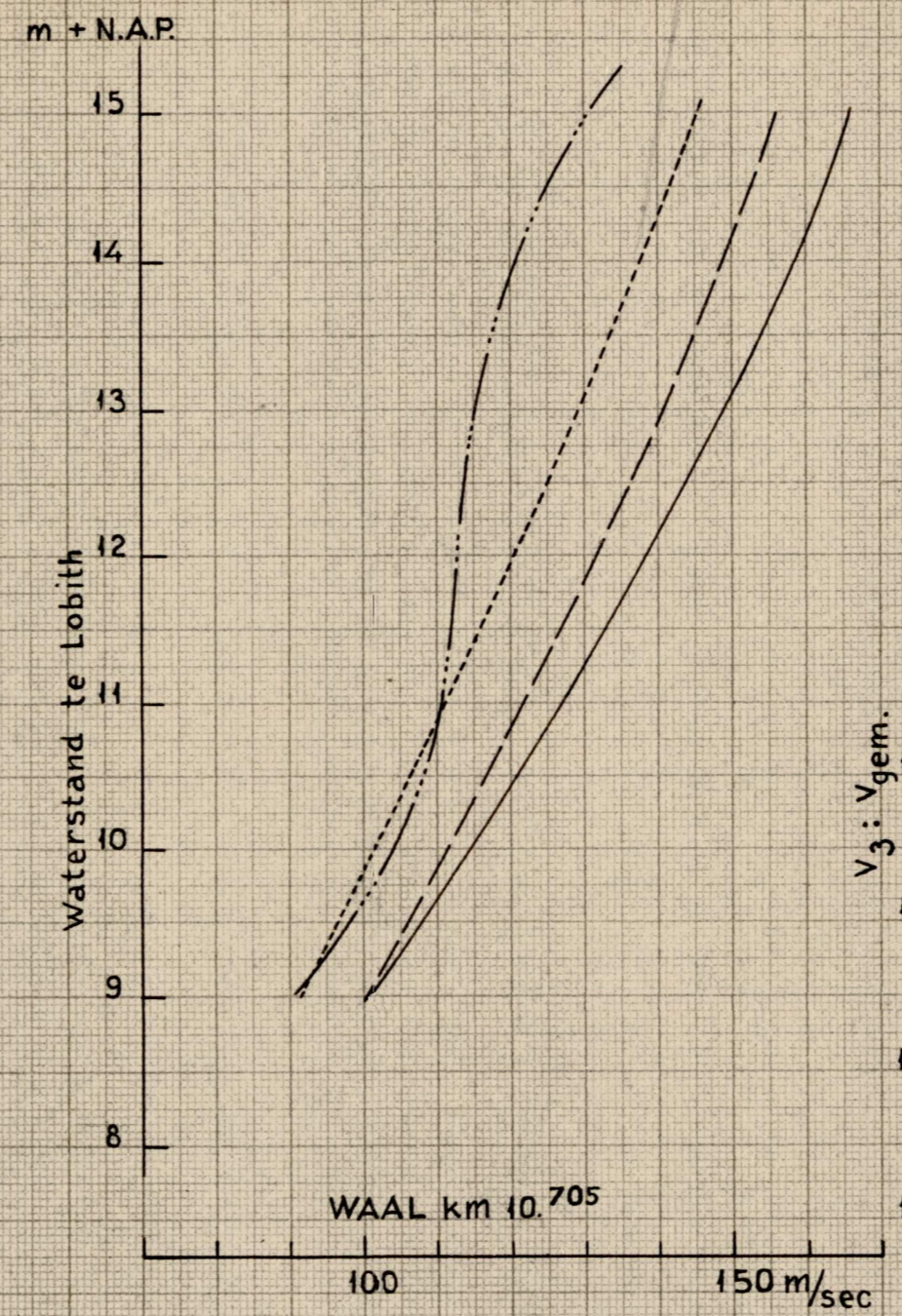
Verband tusschen de snelheid in de bovenste 3m en de gemiddelde snelheid in een verticaal.
