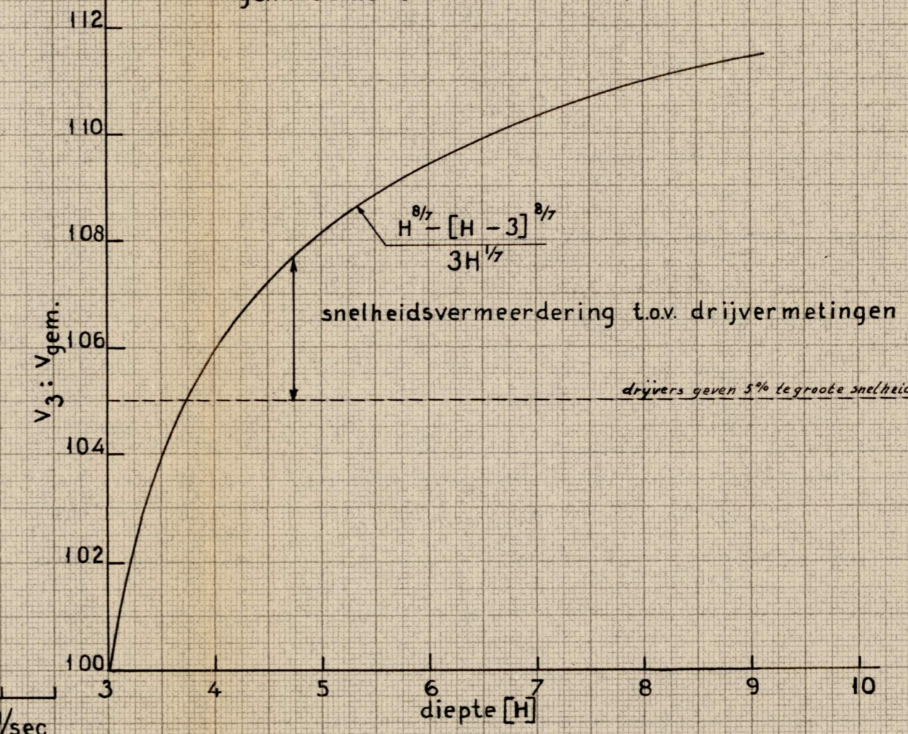
Verband tusschen de snelheid in de bovenste 3m en de gemiddelde snelheid in een verticaal.
