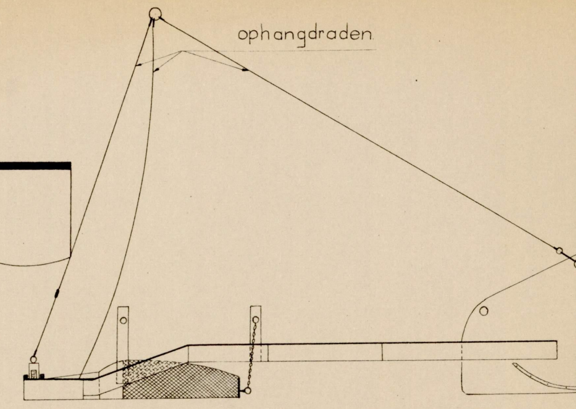
ZUAANZICHT.
