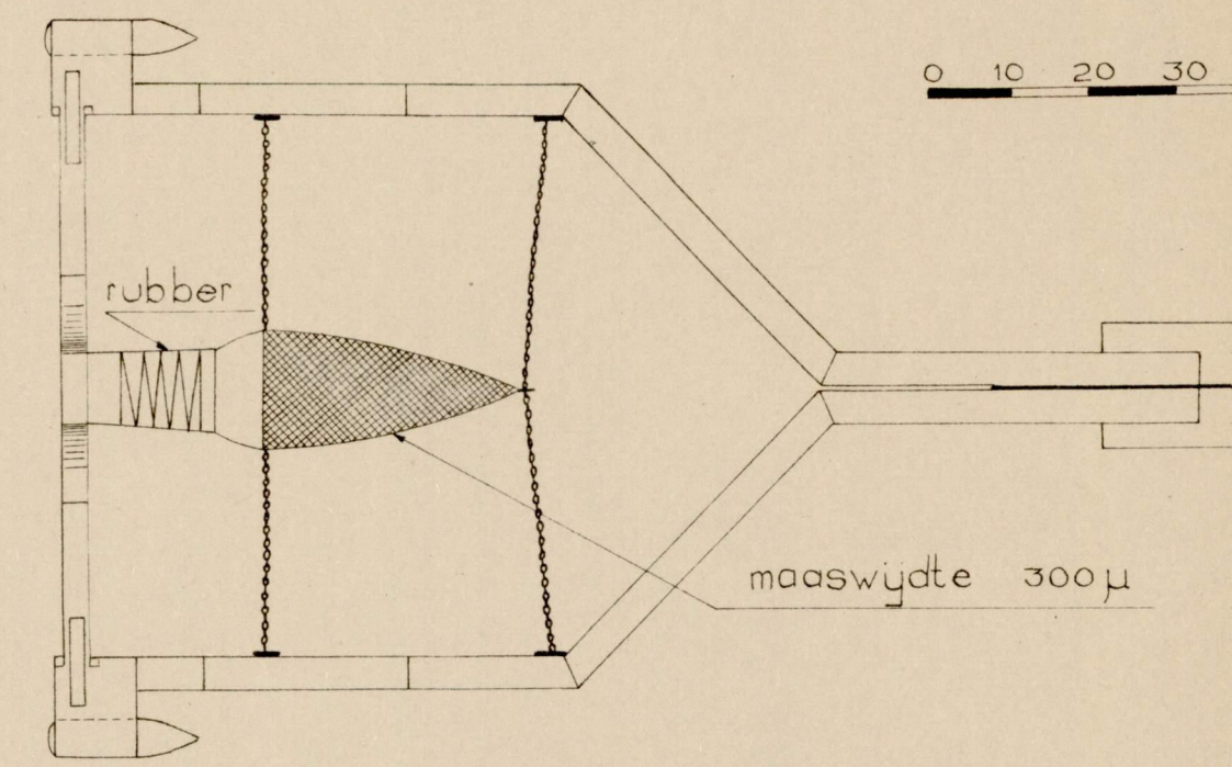
BOVENAANZICHT.
