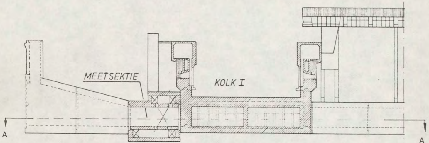
LANGSDOORSNEDE
