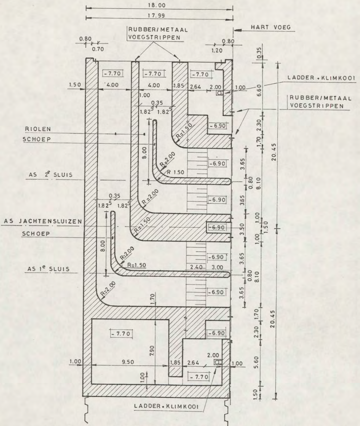
HORizontale Doorsnede D-D Sluishoofd zijpezijde Aantakking riolen onder de tussenvloer
