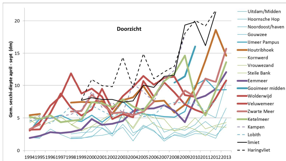
Figuur 5.1. Aanvulling op de grafiek met doorzichtwaarden in het IJsselmeergebied met zomergemiddelde waarden van 2013.
