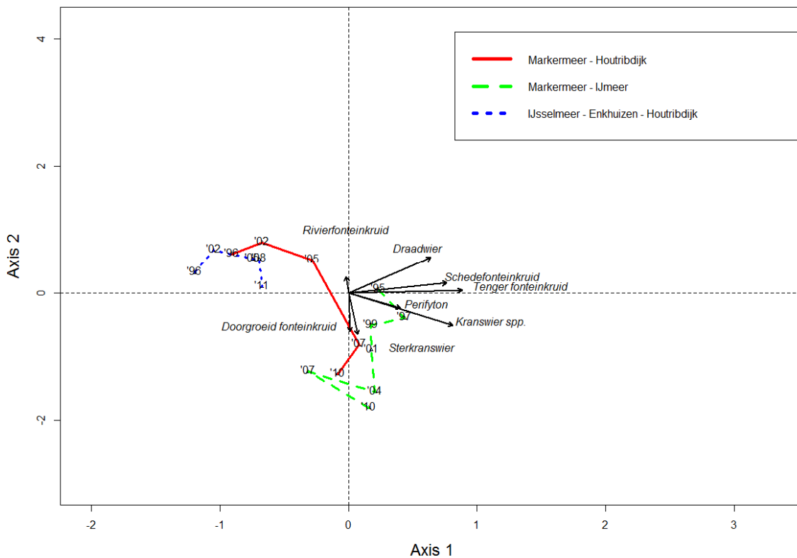
Figuur 3.14. PCA “routes” van de vegetatie in het IJmeer, Markermeer Houtribdijk en IJsselmeer Houtribdijk. De punten vertegenwoordigen jaar-meer combinaties van het gehele IJsselmeergebied. De oudste waarden liggen aan de linker kant van de grafiek.
