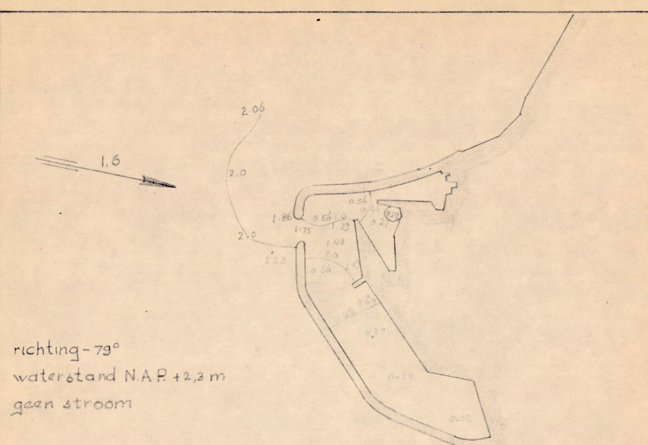
M.167.Figuur 16.5-1.Golfmeting.
