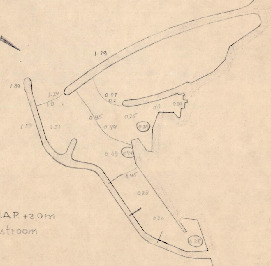
M.167.Figuur 29.512.Golfmeting.
