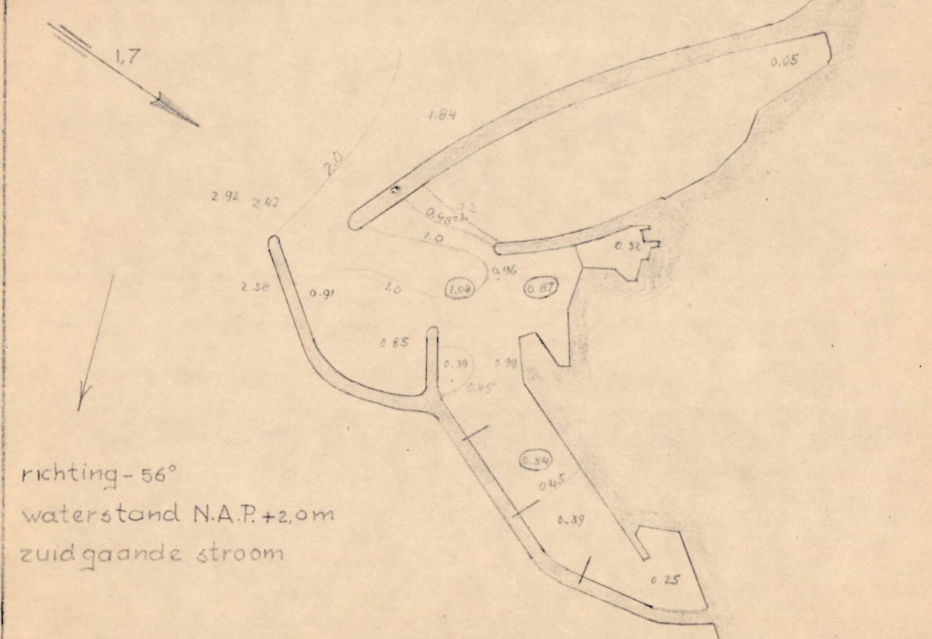
M.167.Figuur 23.56.Golfmeting.
