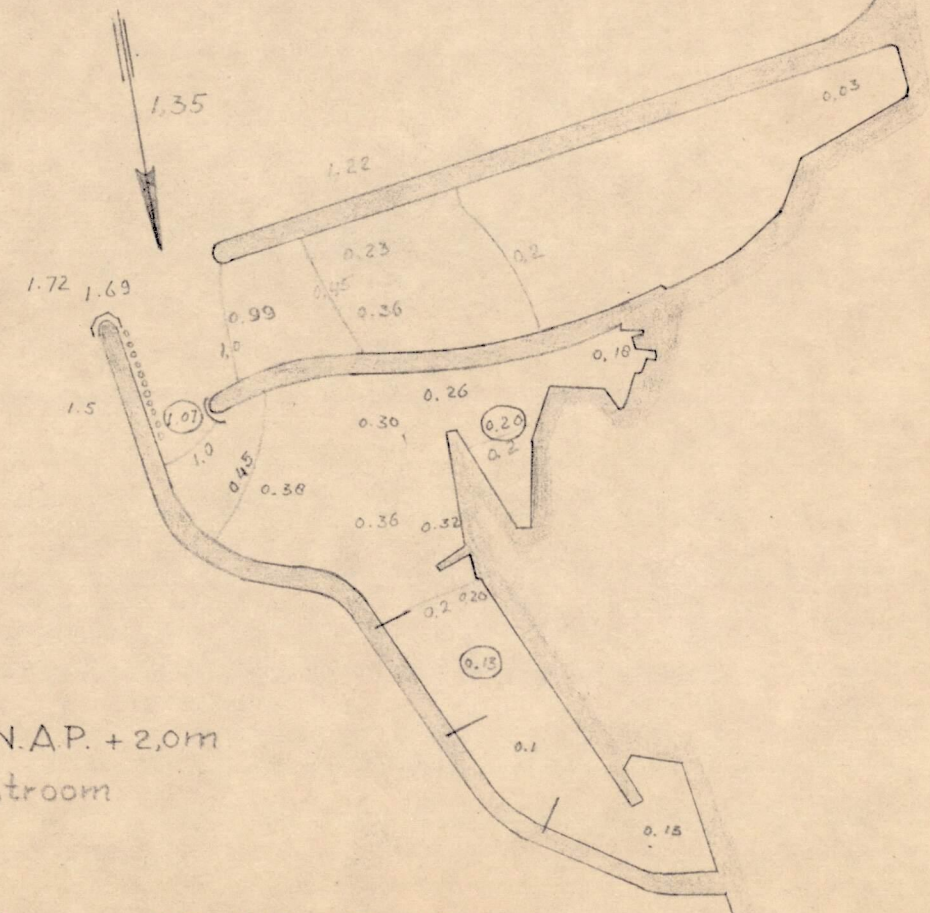
M.167.Figuur 19.52.Golfmeting.
