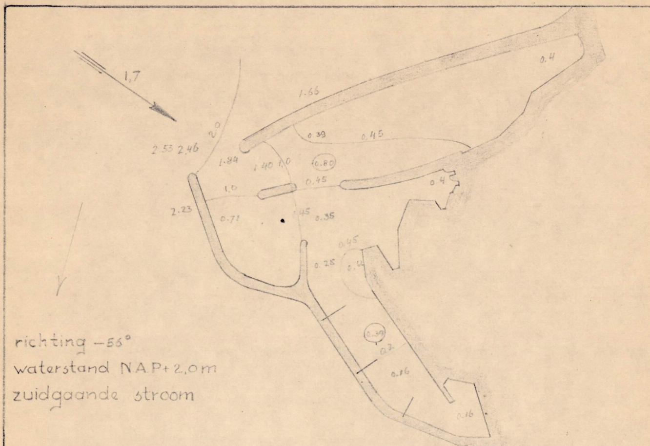
M.167.Figuur 22.55.Golfmeting.
