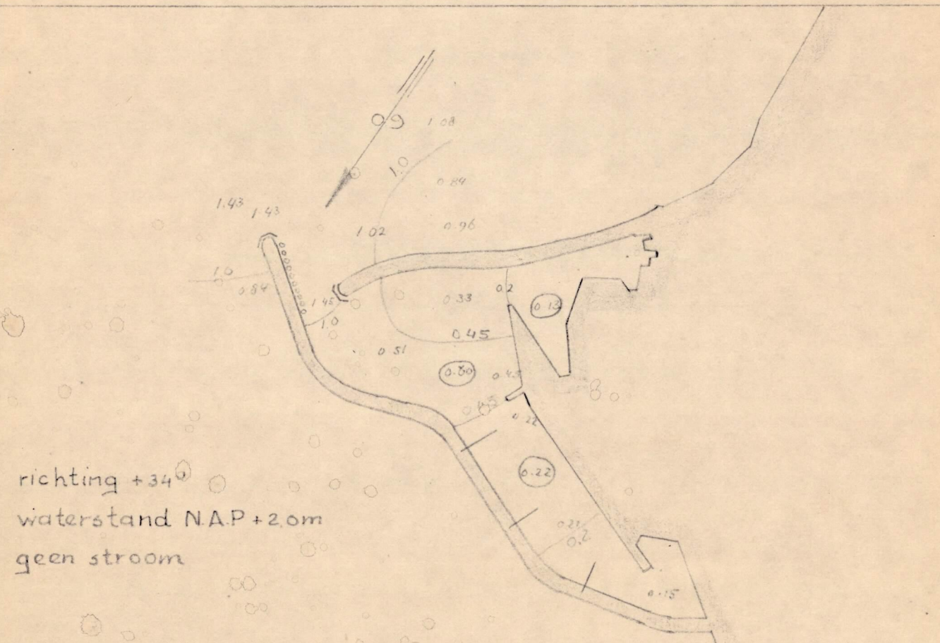
M.167.Figuur 17.51.Golfmeting.
