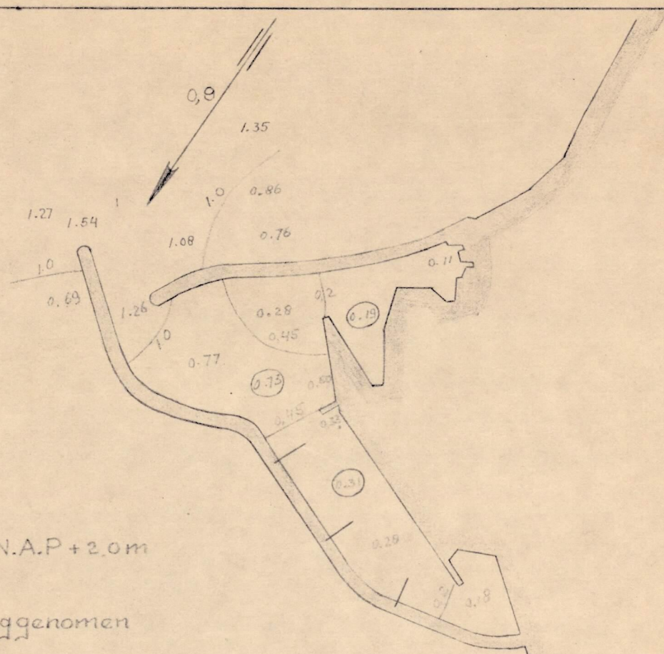
M.167.Figuur 18.51.Golfmeting.
