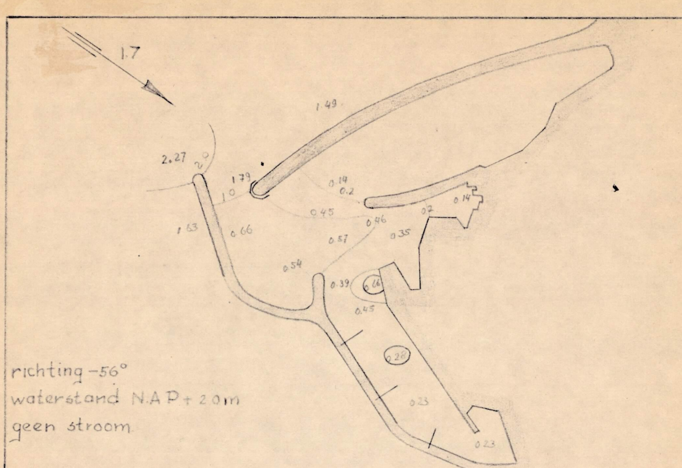
M.167.Figuur 34.517.Golfmeting.
