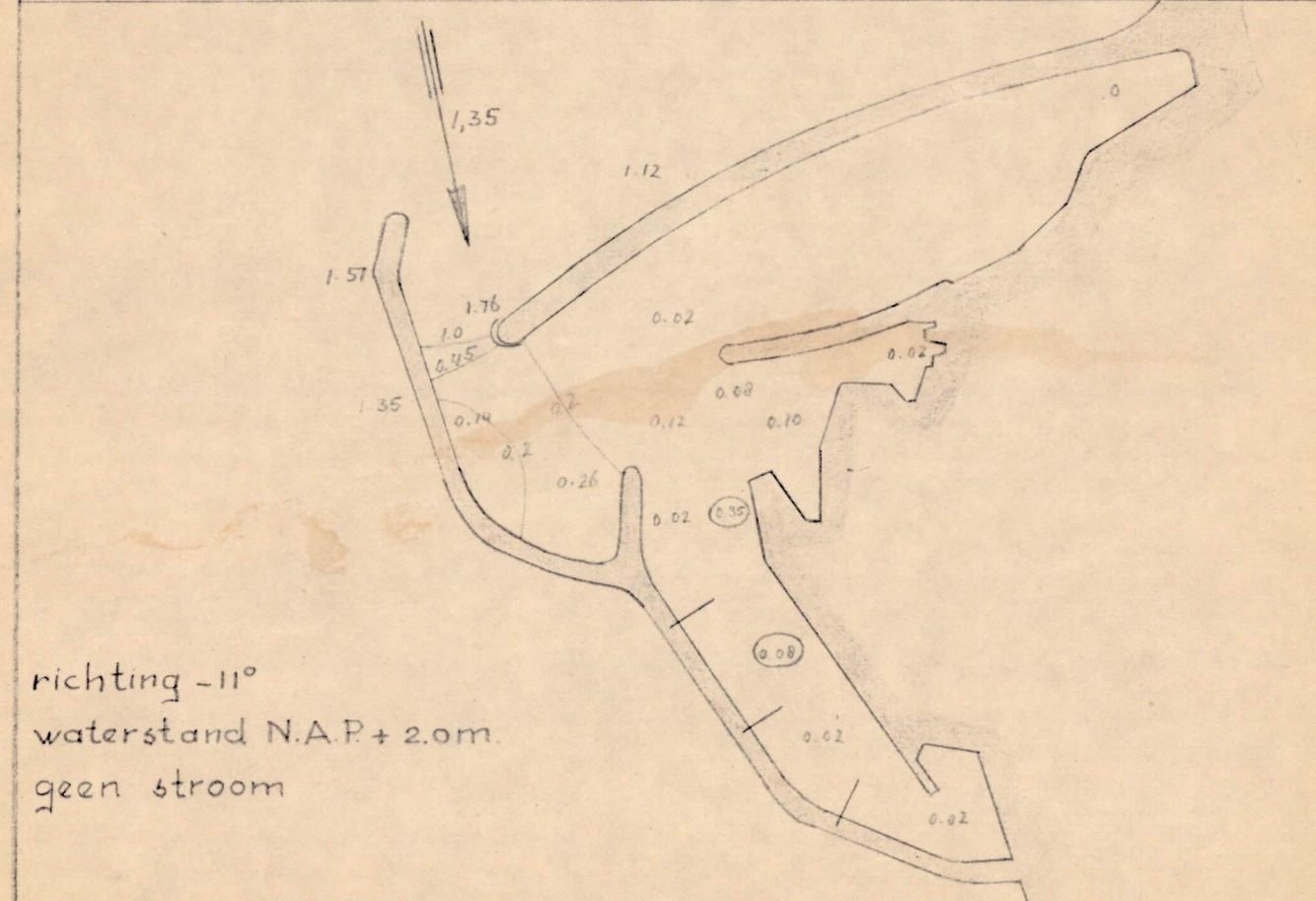
M.167.Figuur 25.58.Golfmeting.
