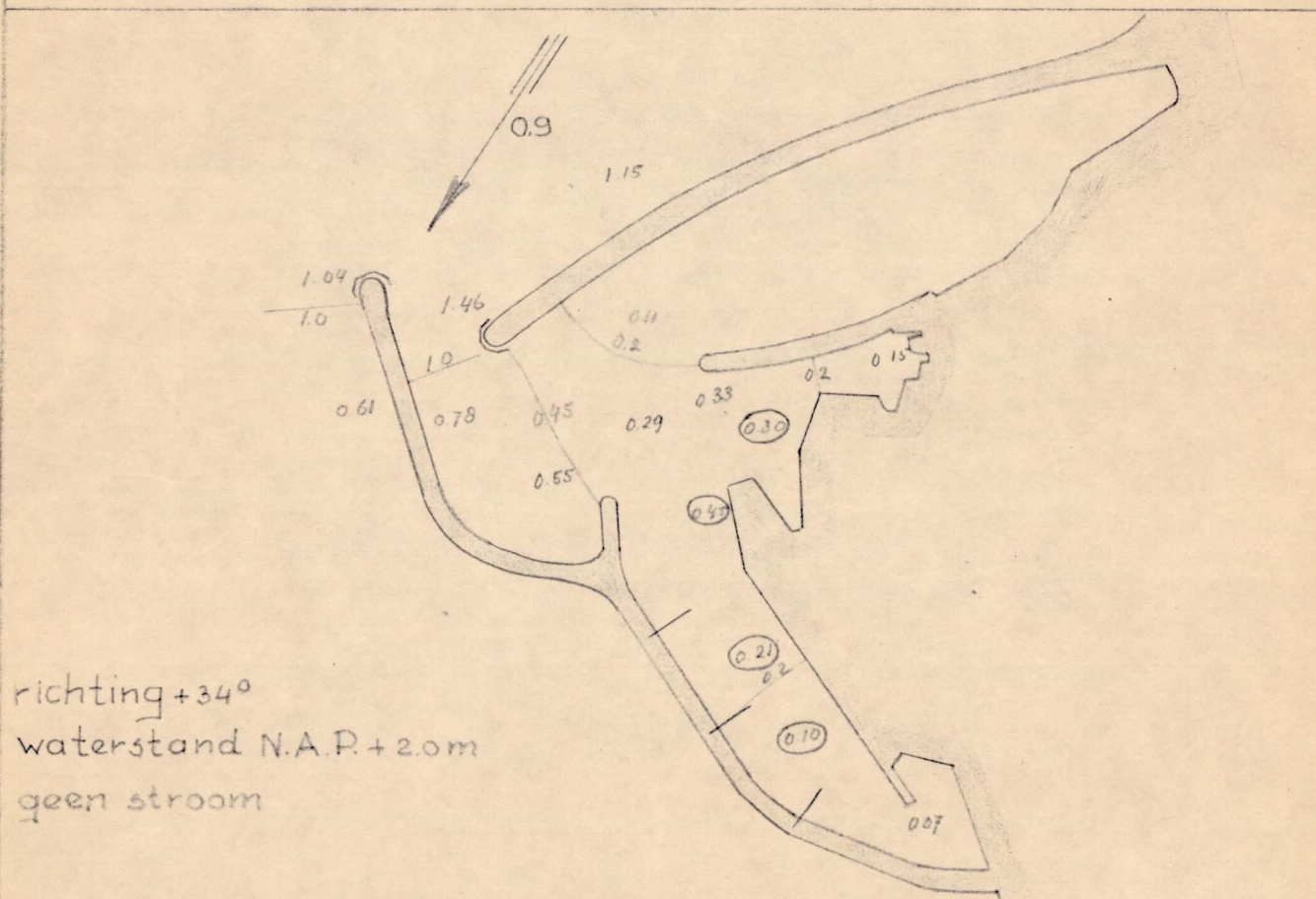
M.167.Figuur 33.516.Golfmeting.
