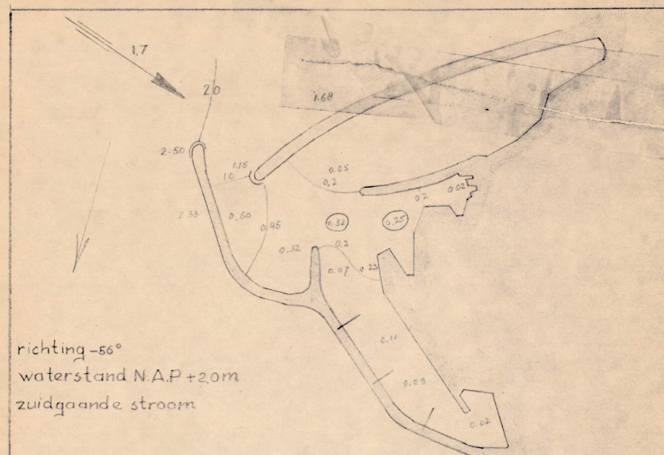
M.167.Figuur 26.59.Golfmeting.
