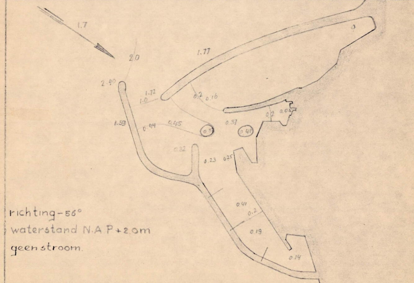
M.167.Figuur 27.510.Golfmeting.
