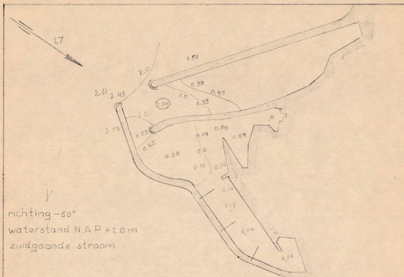
M.167.Figuur 20.53.Golfmeting.
