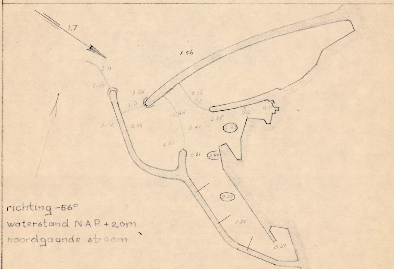
M.167.Figuur 35.518.Golfmeting.
