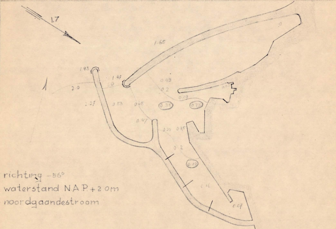
M.167.Figuur 31.514.Golfmeting.
