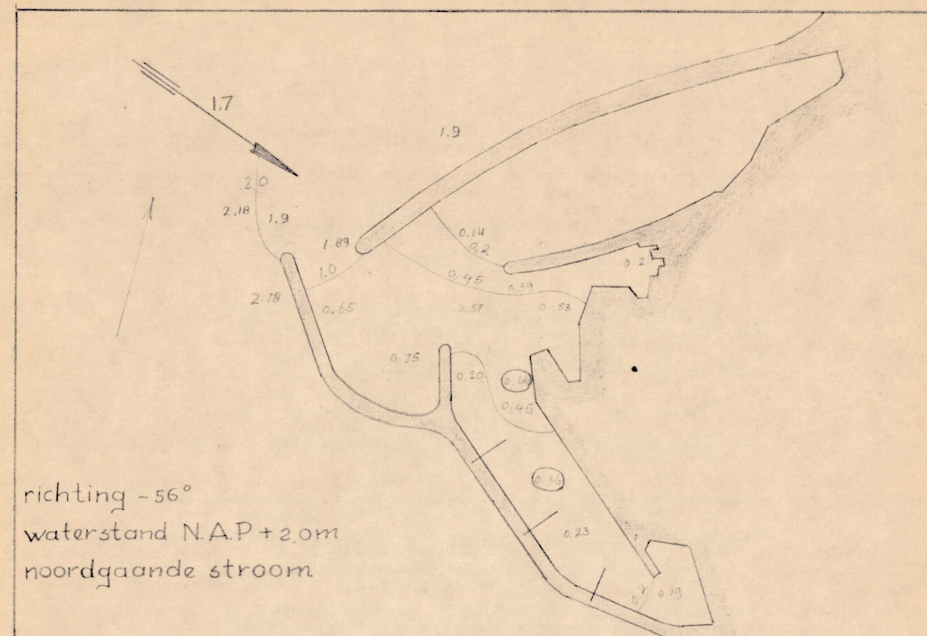
M.167.Figuur 24.57.Golfmeting.
