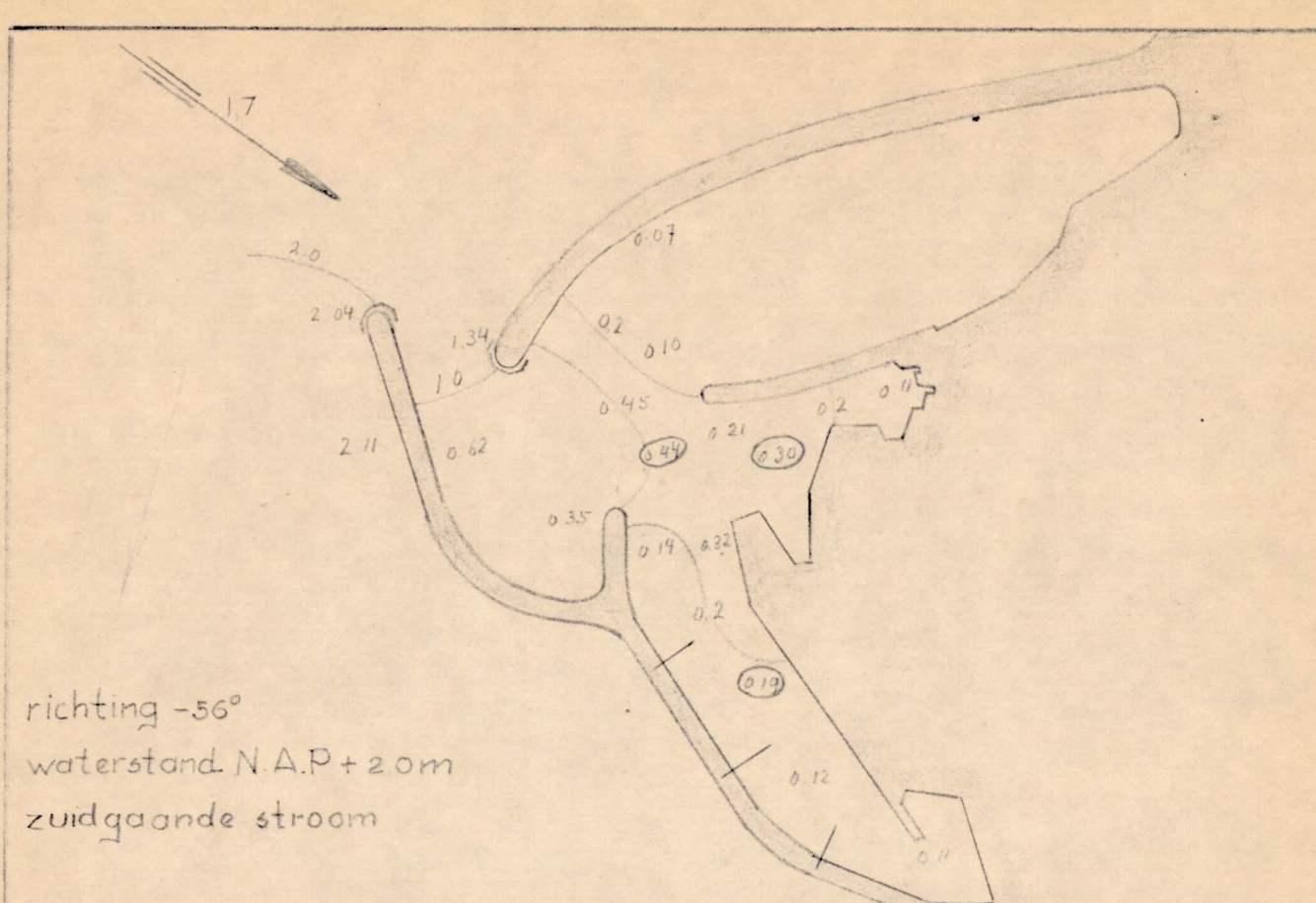
M.167.Figuur 32.515.Golfmeting.
