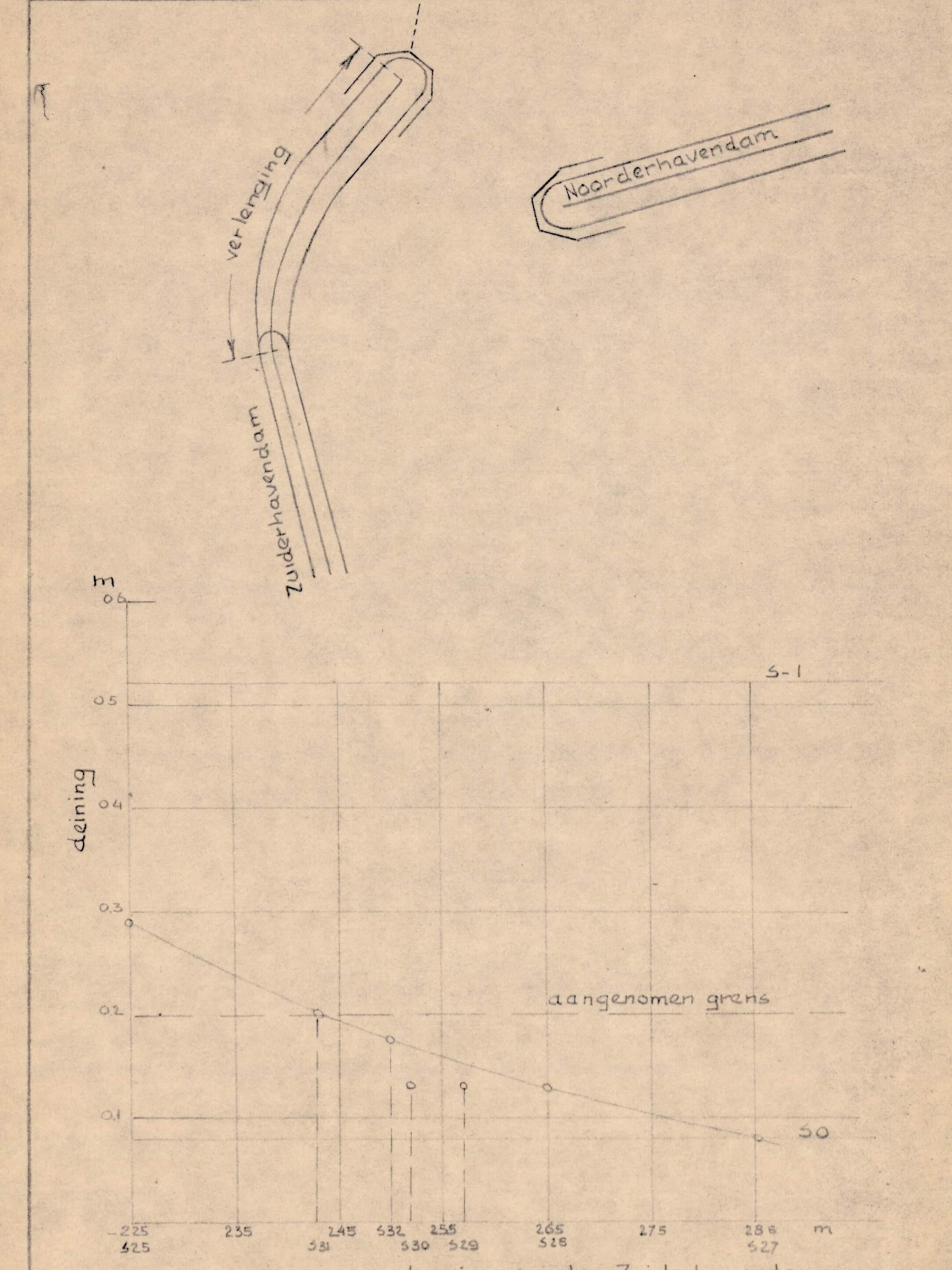
M.167.Fig.42. Hoogte dergolven inde Nieuwe Willemshaven bij verschillende lengten van den Zuiderhavendam.
