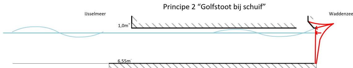
Figuur 3-2: Golfklap type 2: Golfstoot bij schuif. Een deel van de golf weerkaatst en een gedeelte dringt door de koker. Het deel dat doordringt, levert lokaal bij de schuif een golfstoot.
