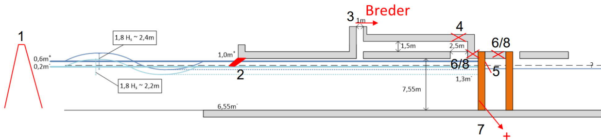
Figuur 5-1: Schetsmatige doorsnede van adaptieve maatregelen
