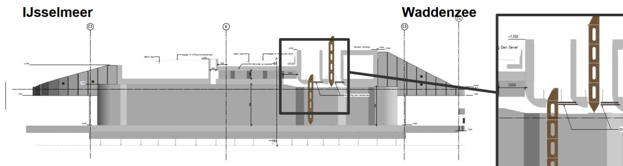
Figuur 2-1: Dwarsdoorsnede schetsontwerp met detail hydraulische vormgeving nabij plafond schuif (Schets VA spuimiddelen)
