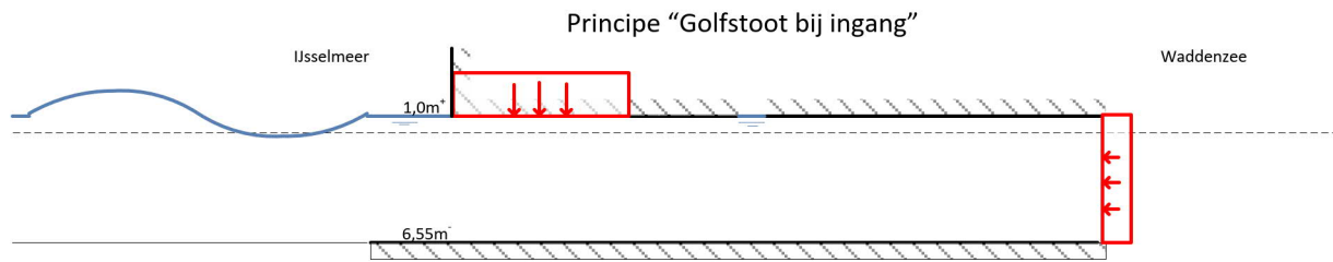
Figuur 3-1: Golfklap type 1: Golfstoot bij ingang. Bij de ingang van de koker aan de IJsselmeerzijde klappt de golf tegen het plafond van de spuisluis. Deze klap levert én een lokale belasting op het plafond, maar zorgt ook voor een drukgolf bij de schuif. Een opening in het plafond van de koker vermindert deze drukstoot op de schuif.
