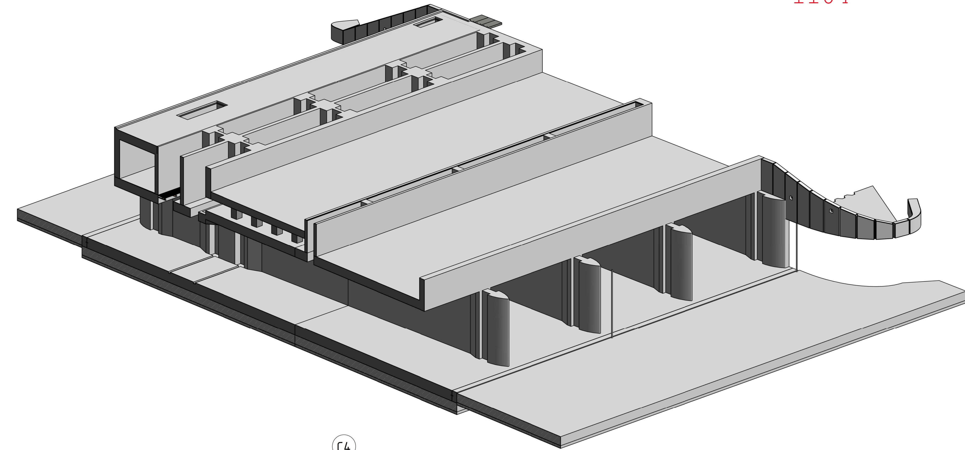
3D overzicht betonwerk Schaal
