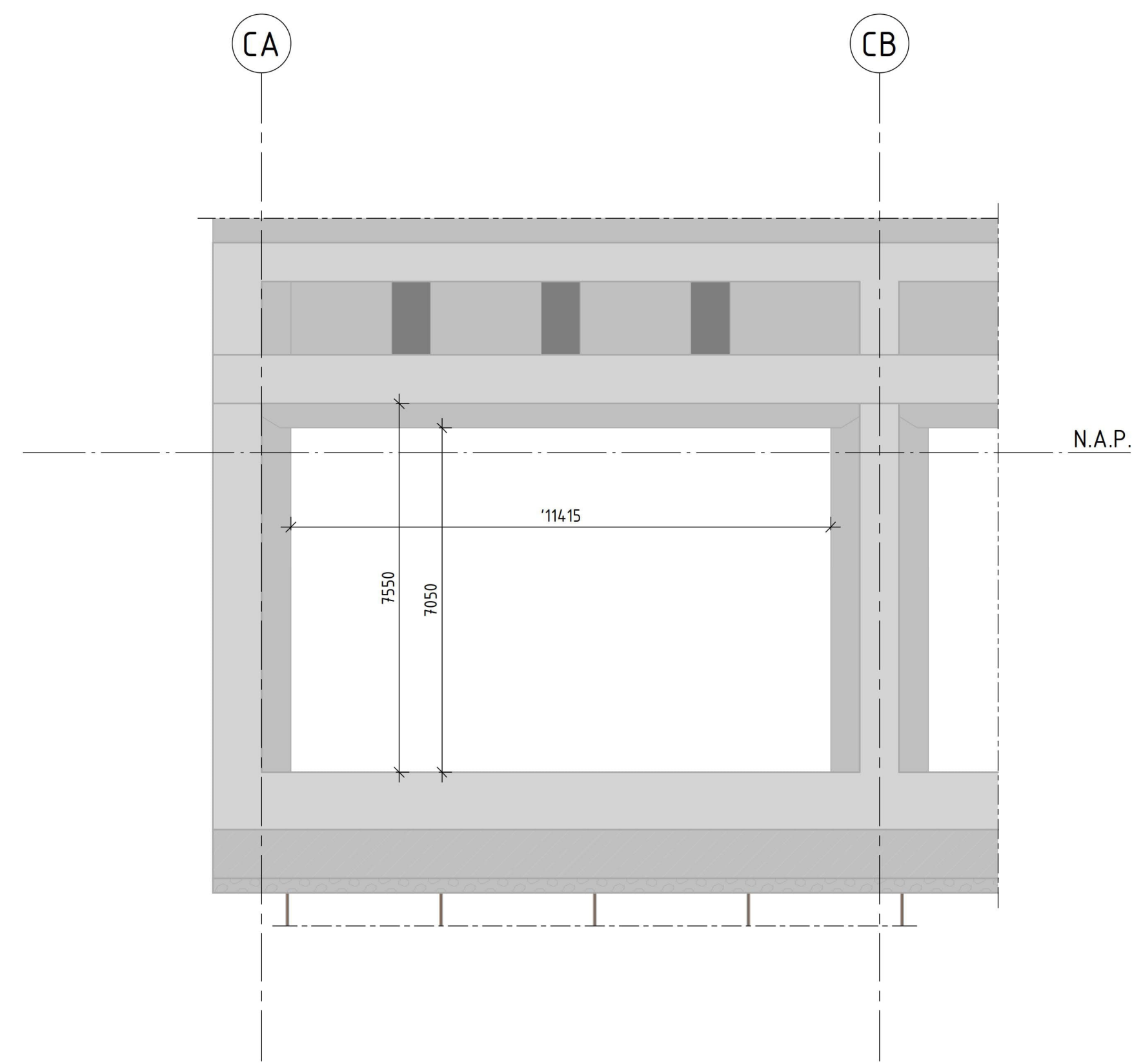
Doorsnede A-A - Aanzicht spuikoker Schaal 1 : 100
