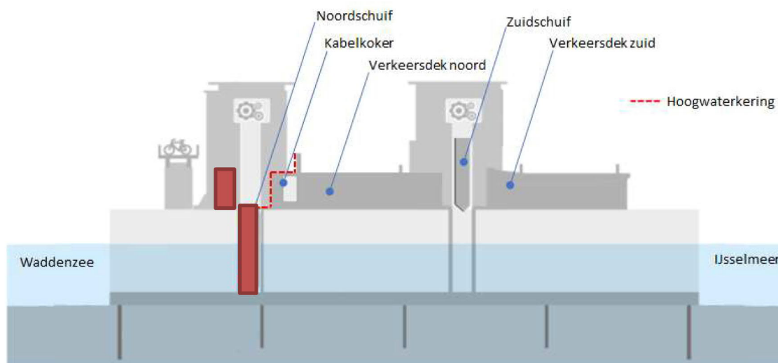
Figuur 1 Doorsnede bestaand spuimiddel over de spuikoker volgens aanbiederontwerp
