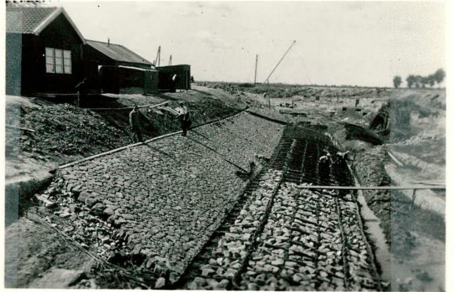
Afgraving "Molenplaats"; aanleg steenglooiing en kraagstukken in den droge; tekst pag. 154.
