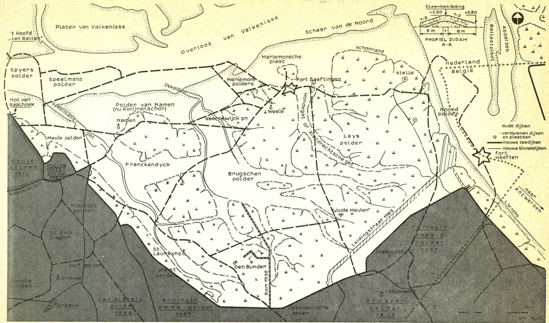
Fig. 24. Het Saftingebied met de v.m. polders (volgens proeve tot reconstructie van Ing K. J. J. Brand te Hulst) en Rijksdam van 1938. Van de verdwenen polders, die merendeels in 1530 overstroomden, verdween als laatste de polder van Namen in 1715. De nieuw bedijkte polders zijn arijs actiet.
