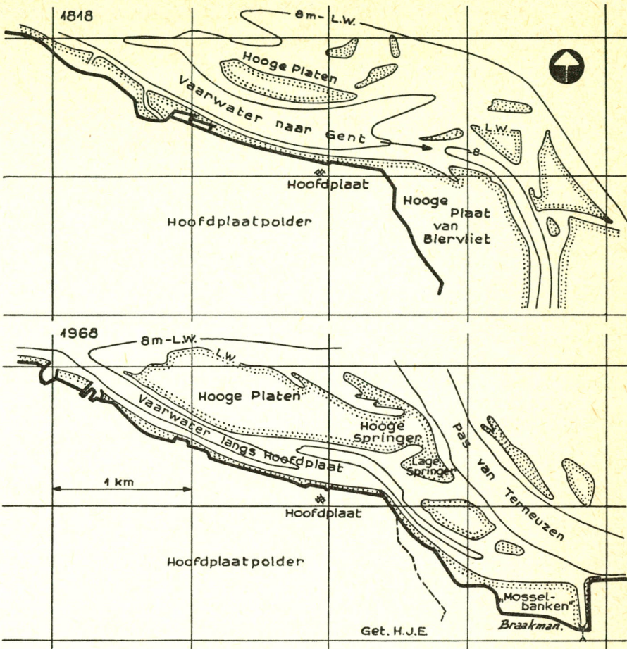
Fig. 30. Situatie van de Hooge Platen in 1818 met het Vaarwater naar Gent en 150 jaar later met de afgedamde Braakman.
