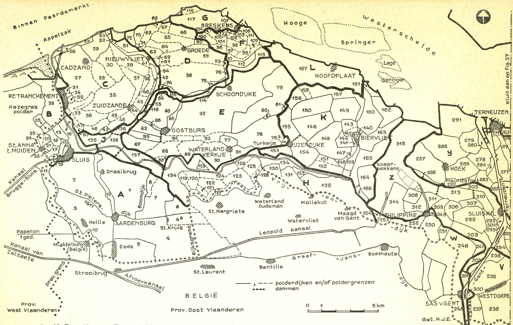
fig. 36. De polders van Zeeuwsch Vlaanderen (westelijk deel). De poldergroepen zijn dikomlijnd en van een letter voorzien volgens de beschrijving in de volgende paragrafen. Voor de nummering der poldernamen zie pag. 79 en 81.
