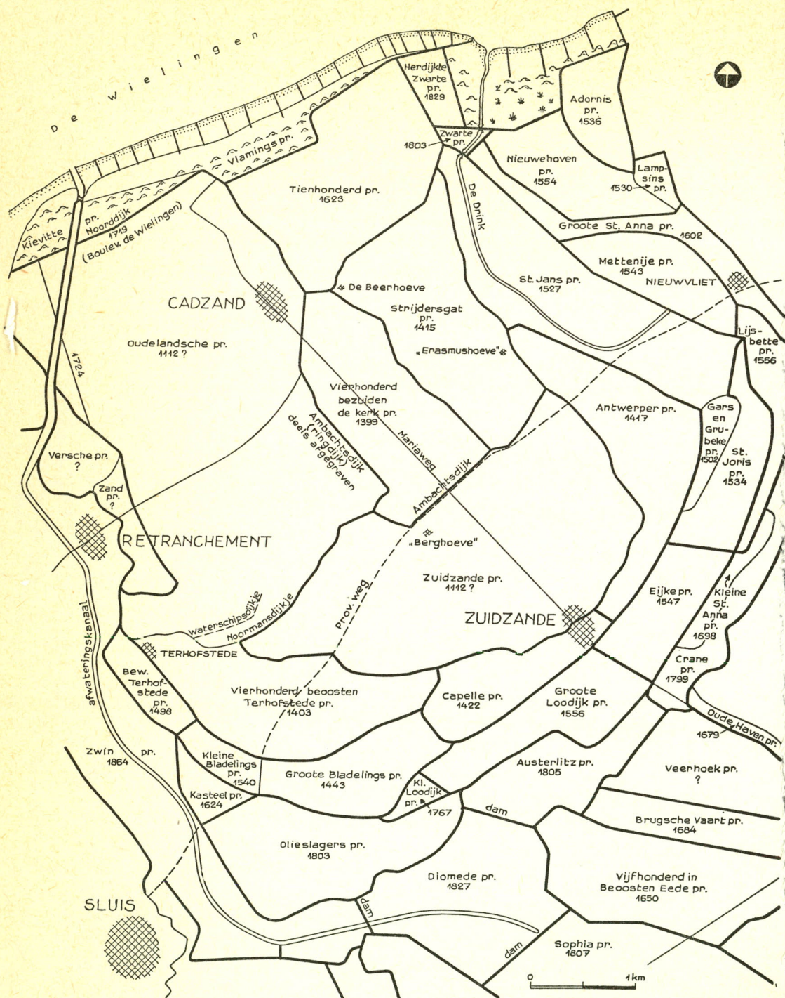
fig. 45. De polders van Cadzand, Zuidzande en Nieuwvliet.
