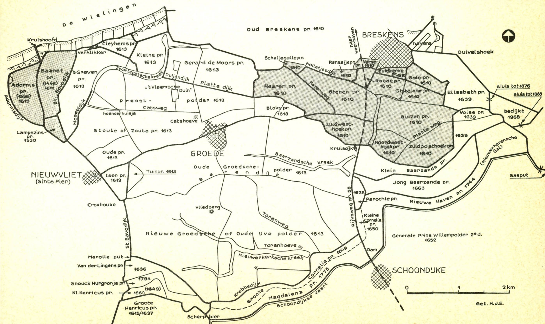
fig. 47. Situatie van de Catspolders c.a. merendeels herdijkt in 1613 en van Groot- en Klein Baarzande c.a. na de inundaties van 1585, merendeels herdijkt in 1610. De grijs getinte gebieden zijn herdijkt in 1610/11 en 1615. De Barendijk was de scheiding tussen de v.m. waterschappen Oude Yvene en Groede.
