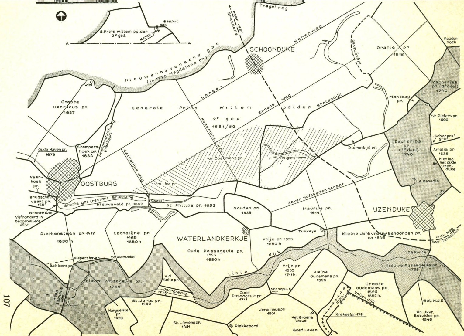
fig. 49. Situatie van de Prins Willempolders. Het v.m. IJzendijke- of Jonkvrouwgat (Zachariaspolders) en de Passageule zijn grijs getint.
