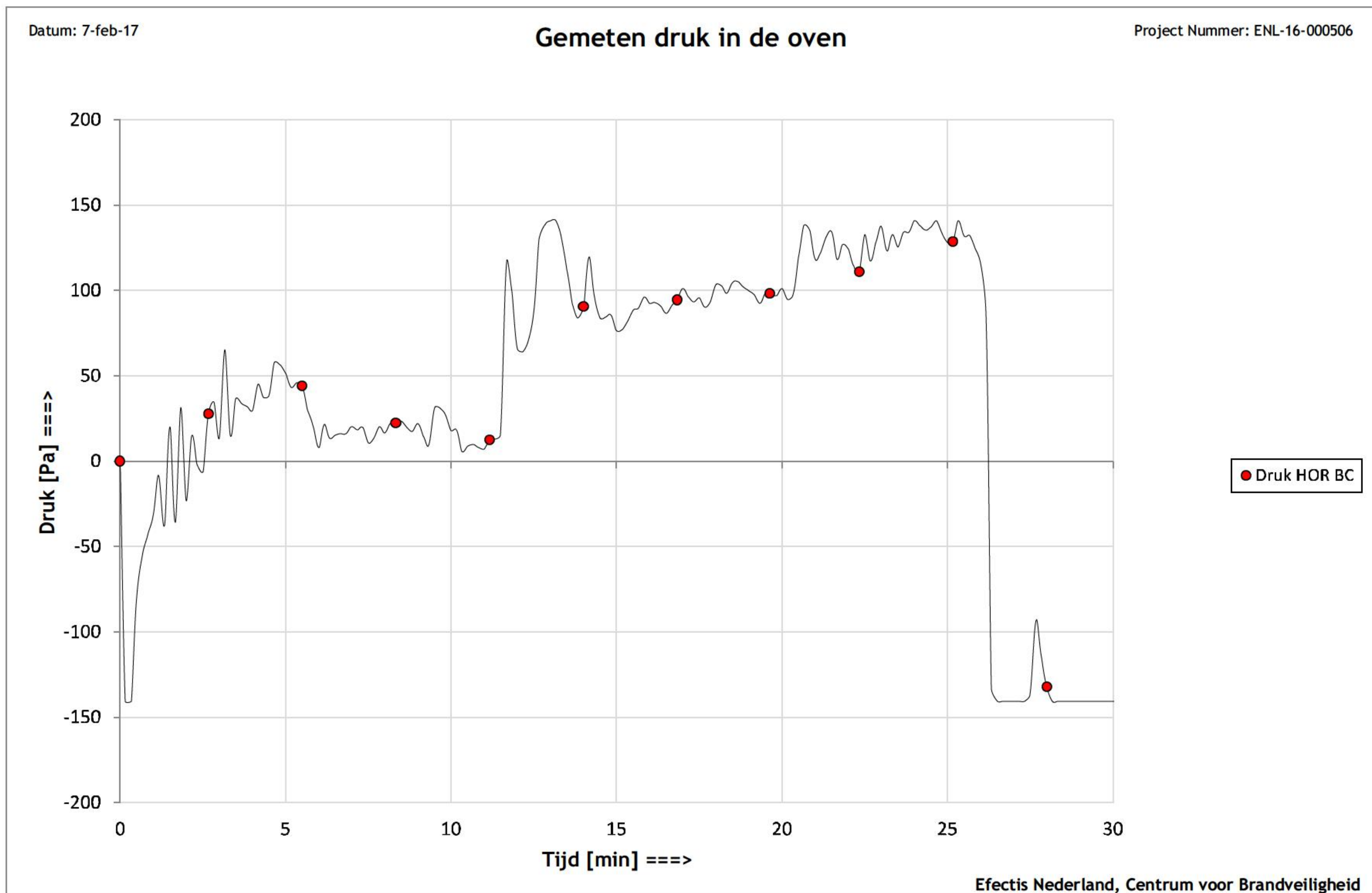
Figuur 2: Druk in de oven (N.B. de metingen na het uitzetten van de oven (T > 26 min) zijn niet relevant meer. Deze zijn voor de volledigheid toegevoegd aan de grafiek.)
