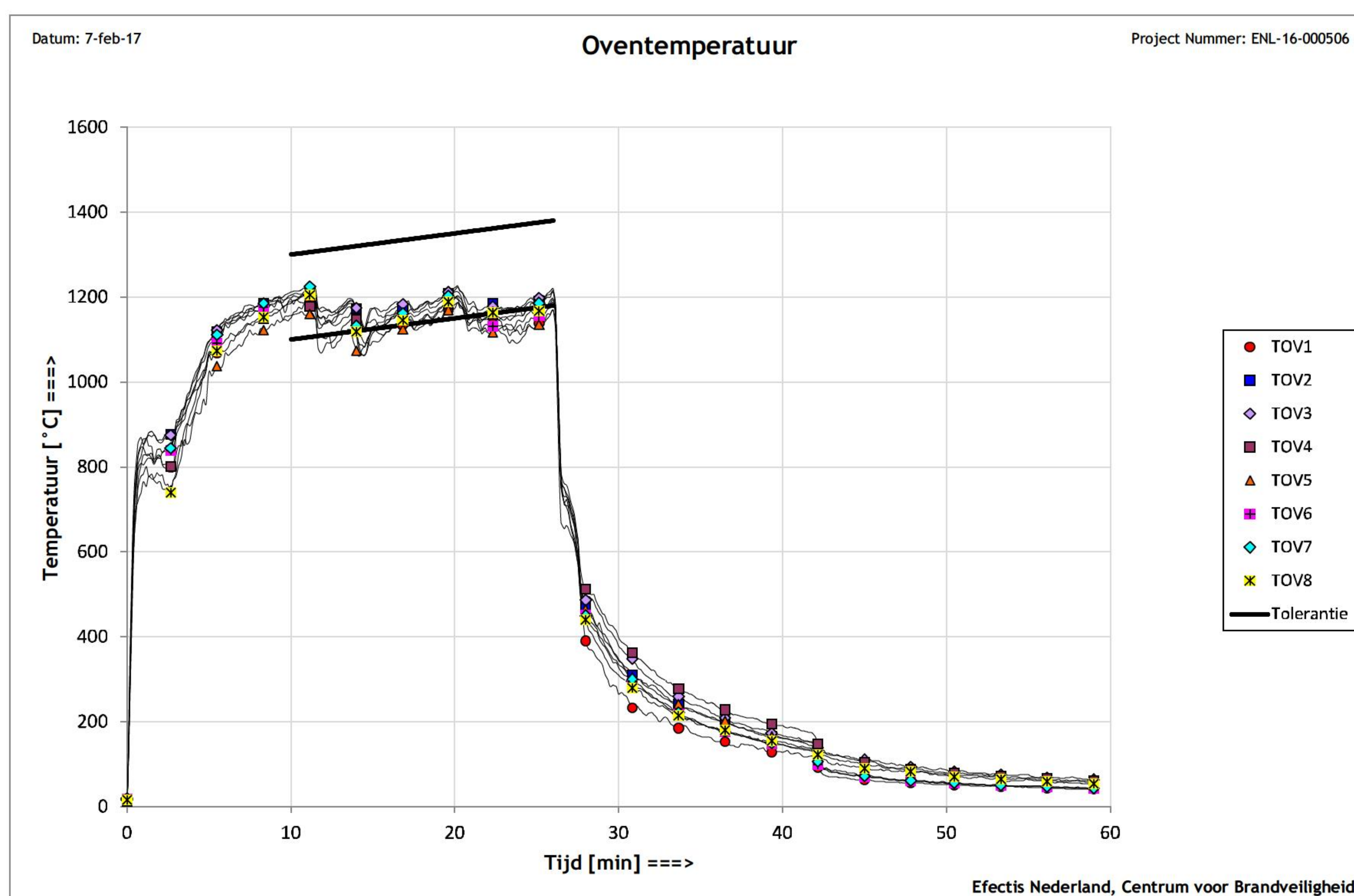
Figuur 1: Oventemperatuur
