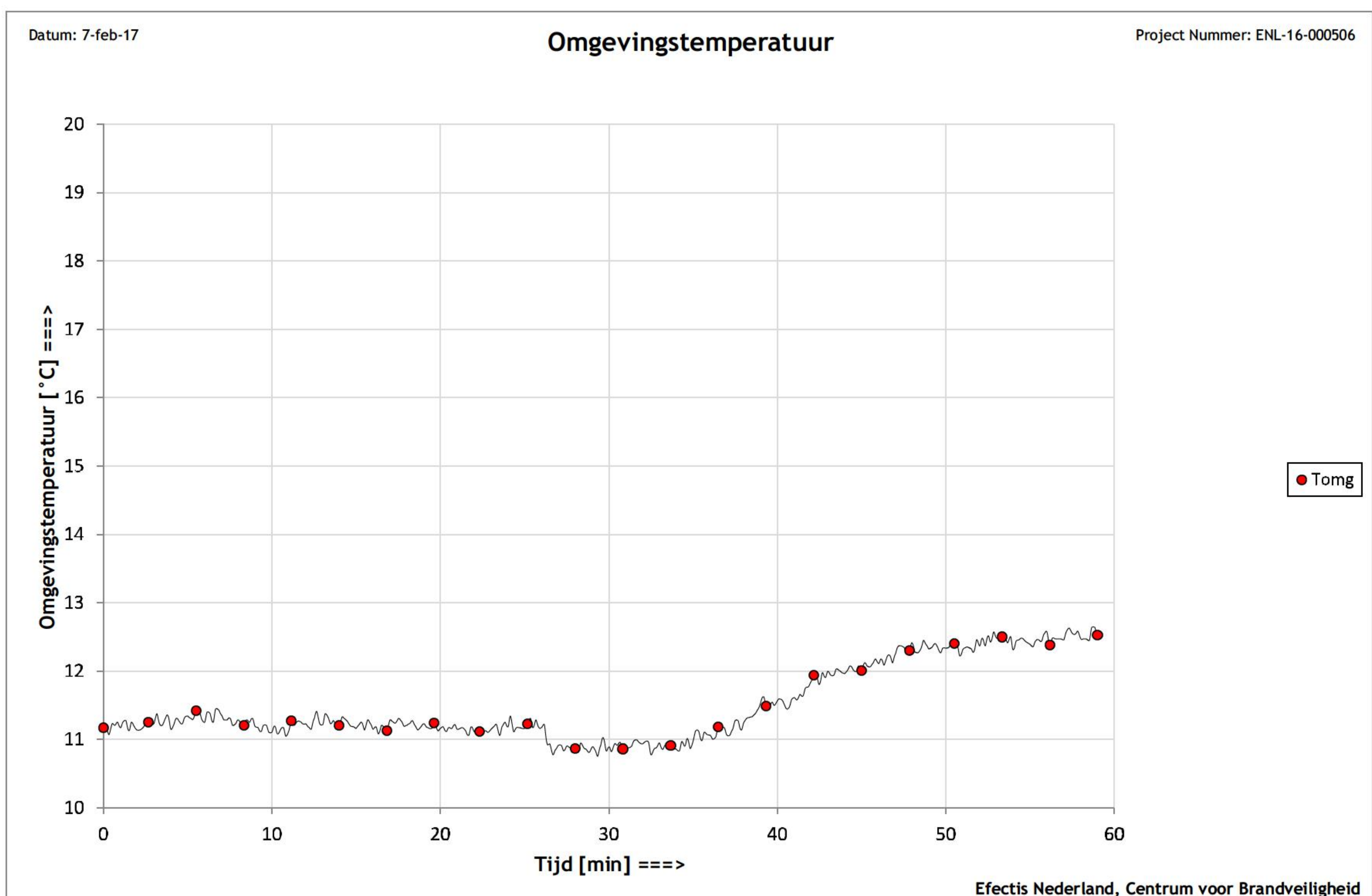
Figuur 3: Omgevingstemperatuur
