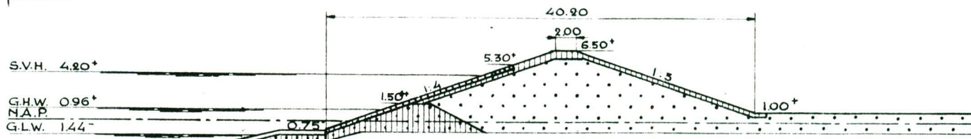
DWARSPROFIEL B-B SCHAAL 1:500
