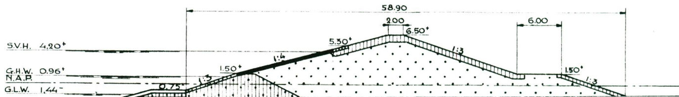
DWARSPROFIEL A-A SCHAAL 1:500
