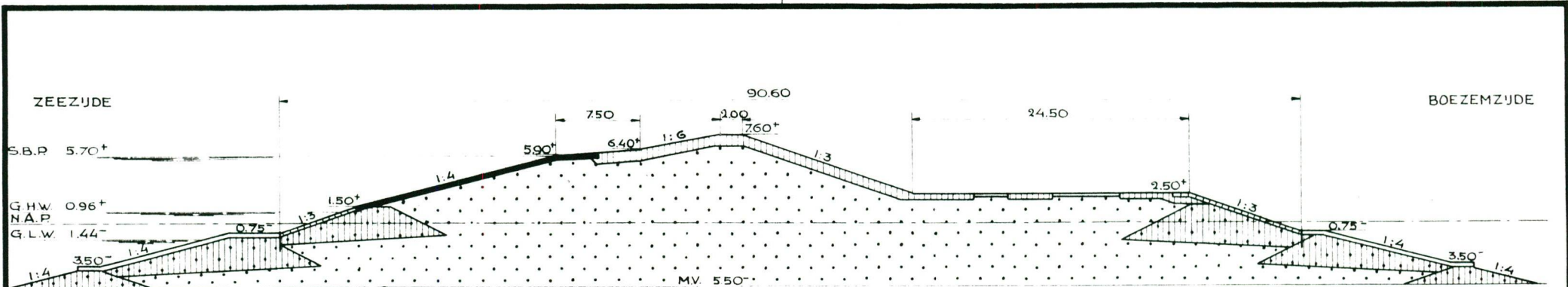
DWARSPROFIEL A-A
