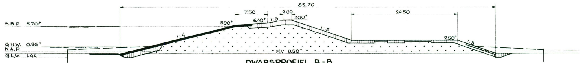
DWARSPROFIEL B-B
