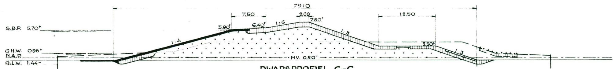
DWARSPROFIEL C-C
