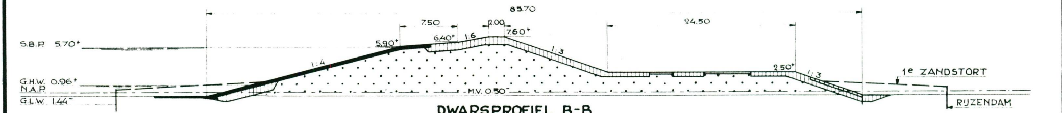
DWARSPROFIEL B-B
