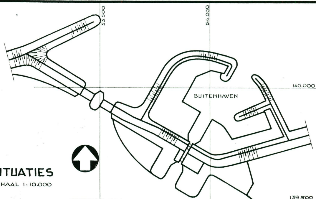
SLUIZEN-HAVENCOMPLEX
