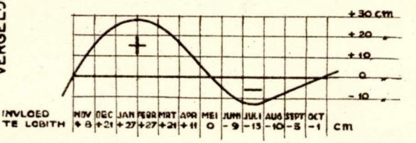
GEMIDDELDE INVLOED VAN RUHR EN LIPPE OP DE WATERSTAND TE LOBITH
