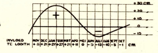
GEMIDDELDE INVLOED VAN RUHR EN LIPPE OP DE WATERSTAND TE LOBITH
