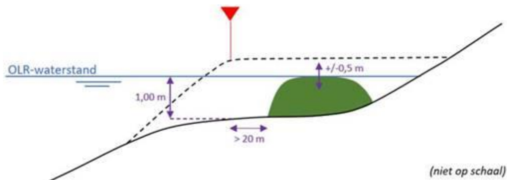
Figuur 3: Dwarsprofiel van principe ontwerp kribvaksuppletie.
