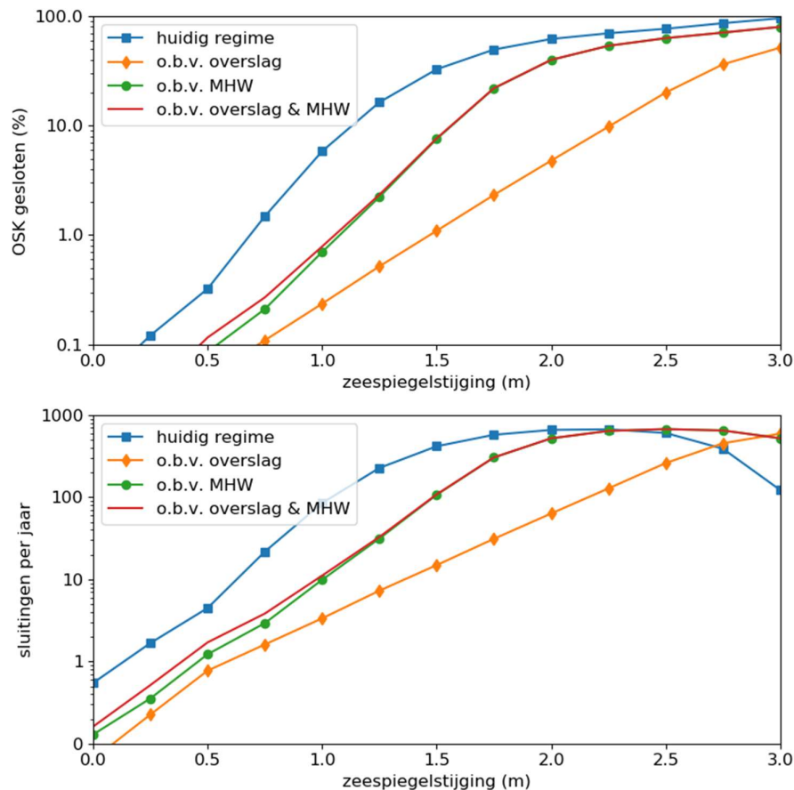
Figuur 5. Percentage van de tijd dat de Oosterscheldekering is gesloten, gebaseerd op criteria voor zee­water­stand (bij het meetpunt Roompot Buiten), overslag­de­biet, MHW en een combinatie daarvan. Sluiten en openen zijn bepaald op basis van een rolling win­dow van 5 uur.
