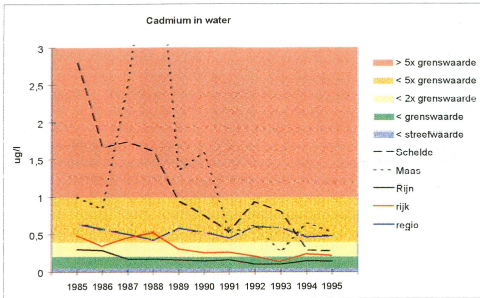
Figuur 3.1.6: Ontwikkeling in de gemiddelde 90-percentielwaarden voor cadmium over de periode 1985-1995 (concentratie in water).
