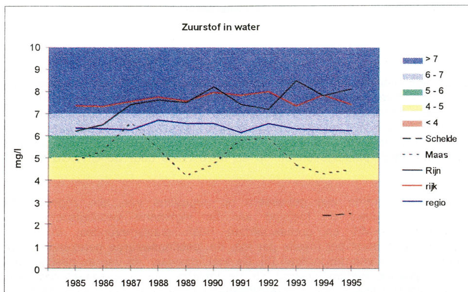
Figuur 3.1.1: Ontwikkeling in de gemiddelde 90-percentielwaarden voor zuurstof over de periode 1985-1995.
