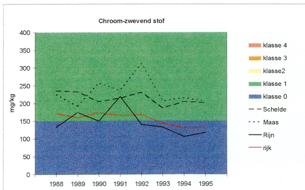
Figuur 3.2.3: Ontwikkeling in de gemiddelde 90-percentielwaarden voor chroom in zwevend stof over de periode 1988-1995..
