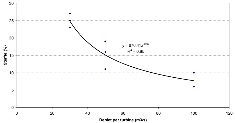
Figuur 1. De sterfte van aal (gemiddelde lengte 60 cm) in relatie tot het debiet per turbine (gegevens op basis van fig. 4.1 in Winter & Jansen 2006). Y = sterftepercentage; X = debiet (m³/s).
