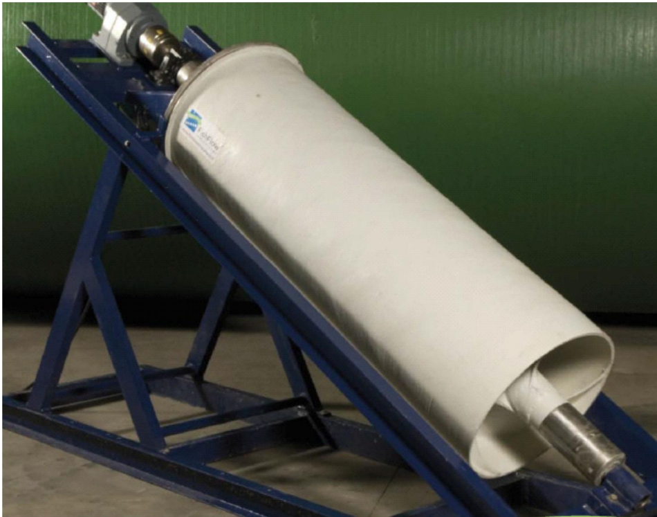
Figuur 10. Vijzelturbine van FFI
