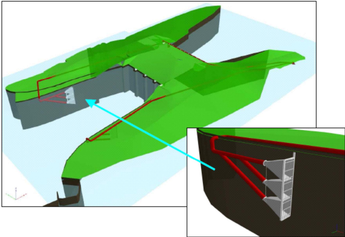
Figuur 1. Visbeschermingssysteem van FishFlow Innovations te Linne
