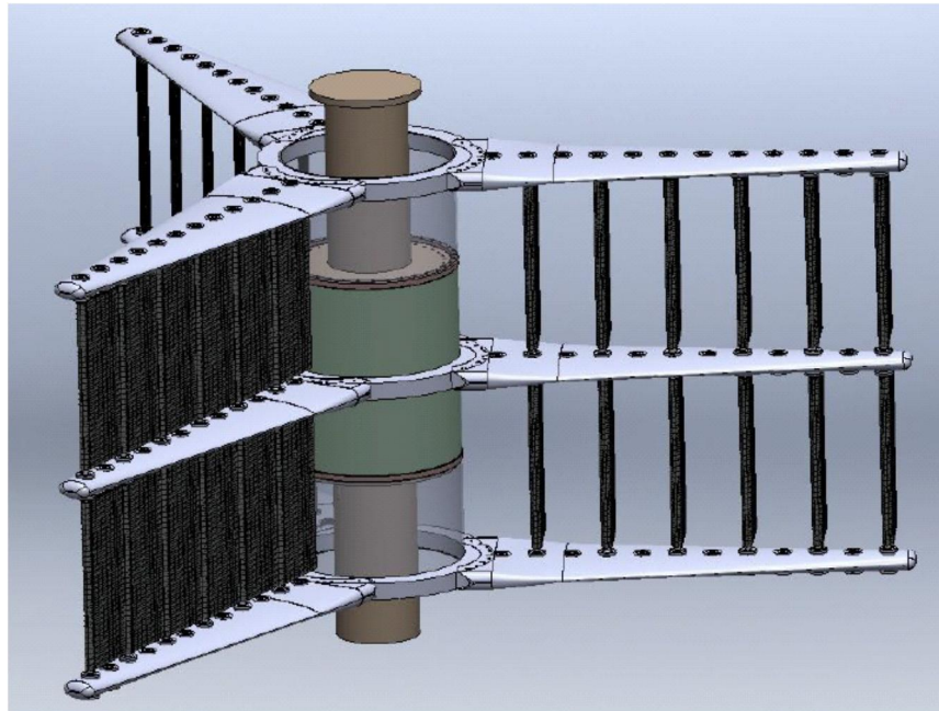
Figuur 11. De Oryon Watermill (voorbeeld: met generator in de as)
