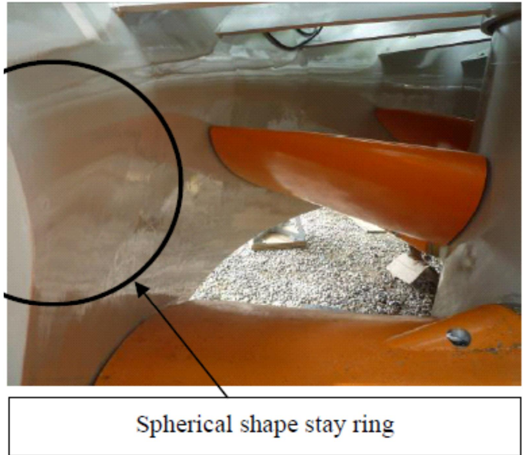
Figuur 9a. VLH turbine met sferische buitenring
