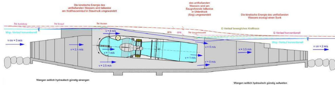
Figuur 6. De submarine centrale
