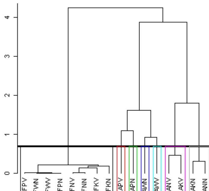
Figuur 22: Cluster dendrogram met \log(x+1) getransformeerde aantallen van de 15 meest abundantste soorten gevangen met ankerkuil en schietfuiken in de Zeeschelde (voor- en najaar 2011)
