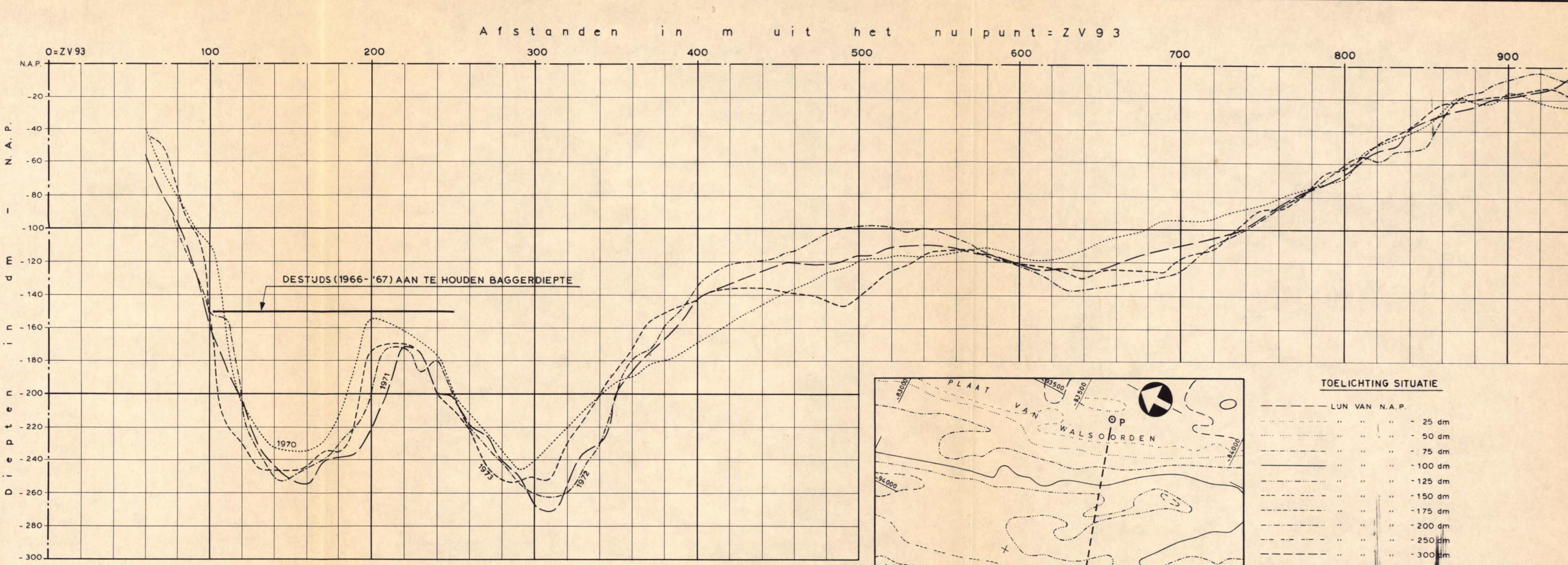
TOELICHTING PROFIELEN DE PROFIELEN ZIJN SAMENGESTELD NAAR LODINGEN RW STUDIEDIENST VLISSINGEN
