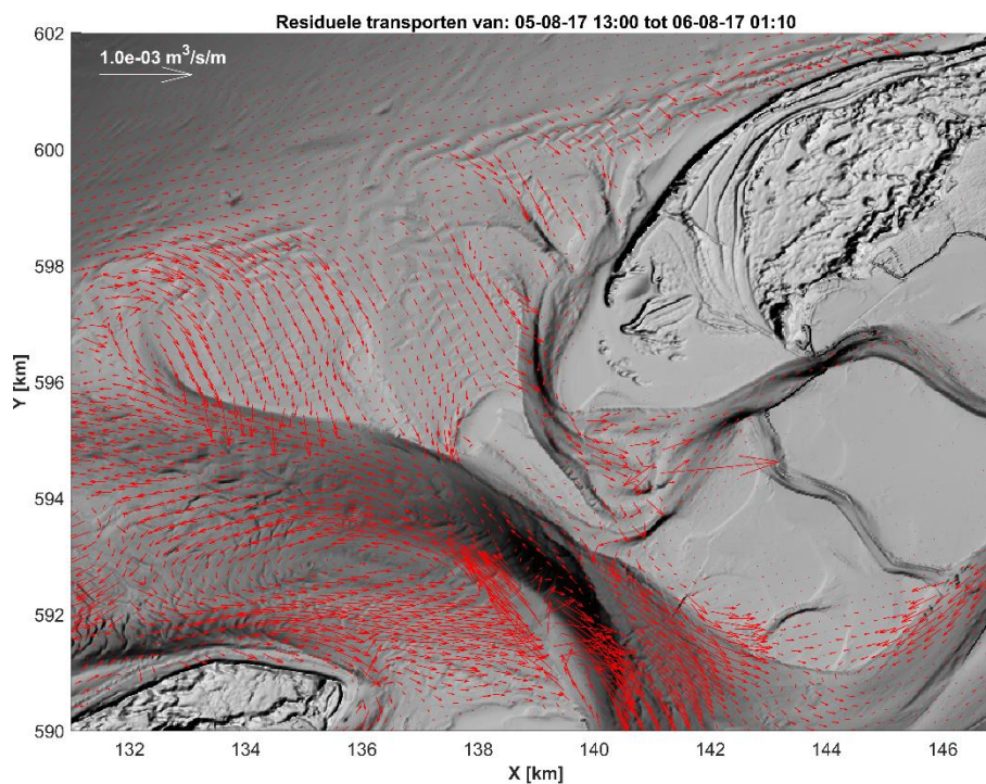
Figuur 6-4 Residuele transporten over het morfologische getij voor het T0 model voor het gewogen gemiddelde van de 4 golfcondities.
