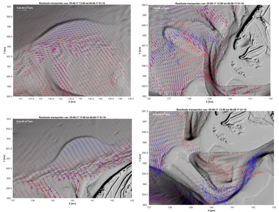
Figuur 6-11 Residuele transporten van de suppletie (blauw) ten opzichte van de T0 situatie (rood) ingezoomd per suppletielocatie. Linksboven: suppletie 1, Rechtsboven: suppletie 2, Linksonder: Suppletie 3, Rechtsonder: Suppletie 4.
