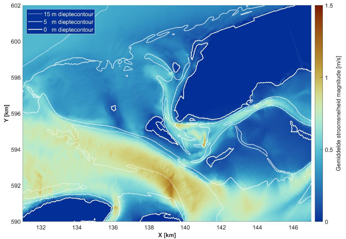
Figuur A-10 Gemiddelde snelheidsmagnitudo van het morfologische getij voor supplementvariant 1
