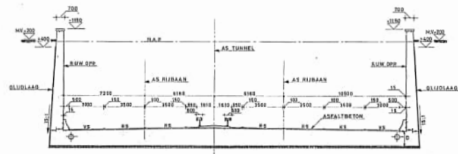
DOORSNEDE B-B
