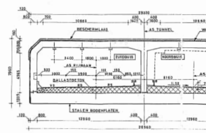
DOORSNEDE C-C
