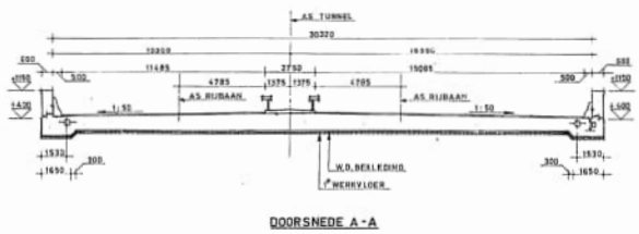
DOORSNEDE A-A
