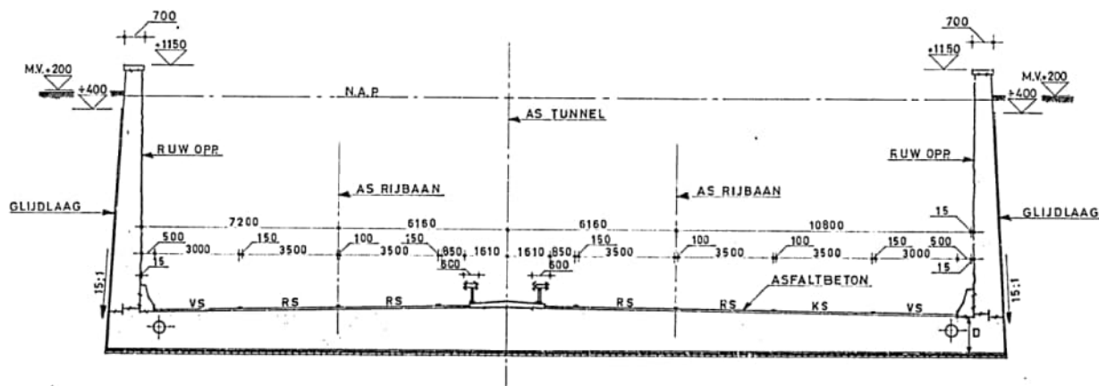
DOORSNEDE B - B
