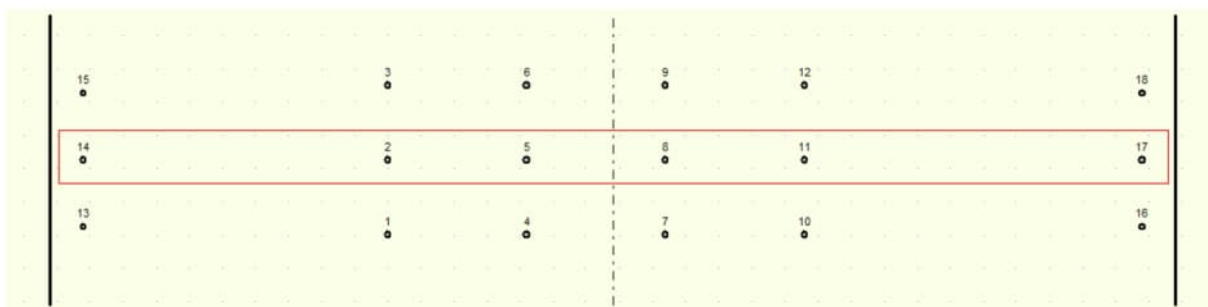
Figuur 7 Invoer palen in D-Foundations o.b.v. palenplan moot 26
