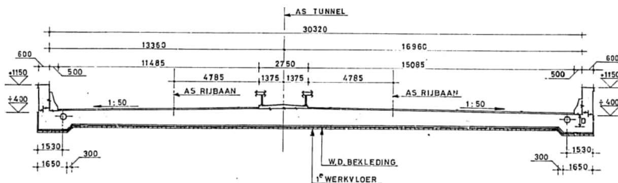
DOORSNEDE A - A
