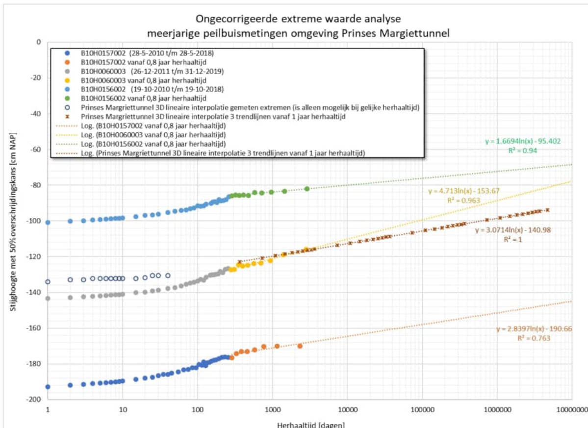
Figuur 6 Extreme waarde analyse op langjarige peilbuiswaarnemingen en 3D interpolatie van waarden ter plaatse van de Prinses Margriettunnel
