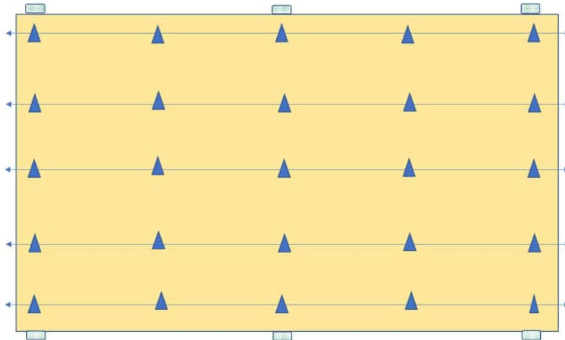
Figuur 1 Overzicht meetpunten voor deformatie bepaling (driehoeken) en voor het vaststellen van holle ruimten onder de vloer (rechthoeken). De pijlpunten links en rechts geven de posities aan waar langs een verticaal op vier hoogtes de vervorming (de uitwijking van of naar de weg-as) van de wand wordt gemeten.
