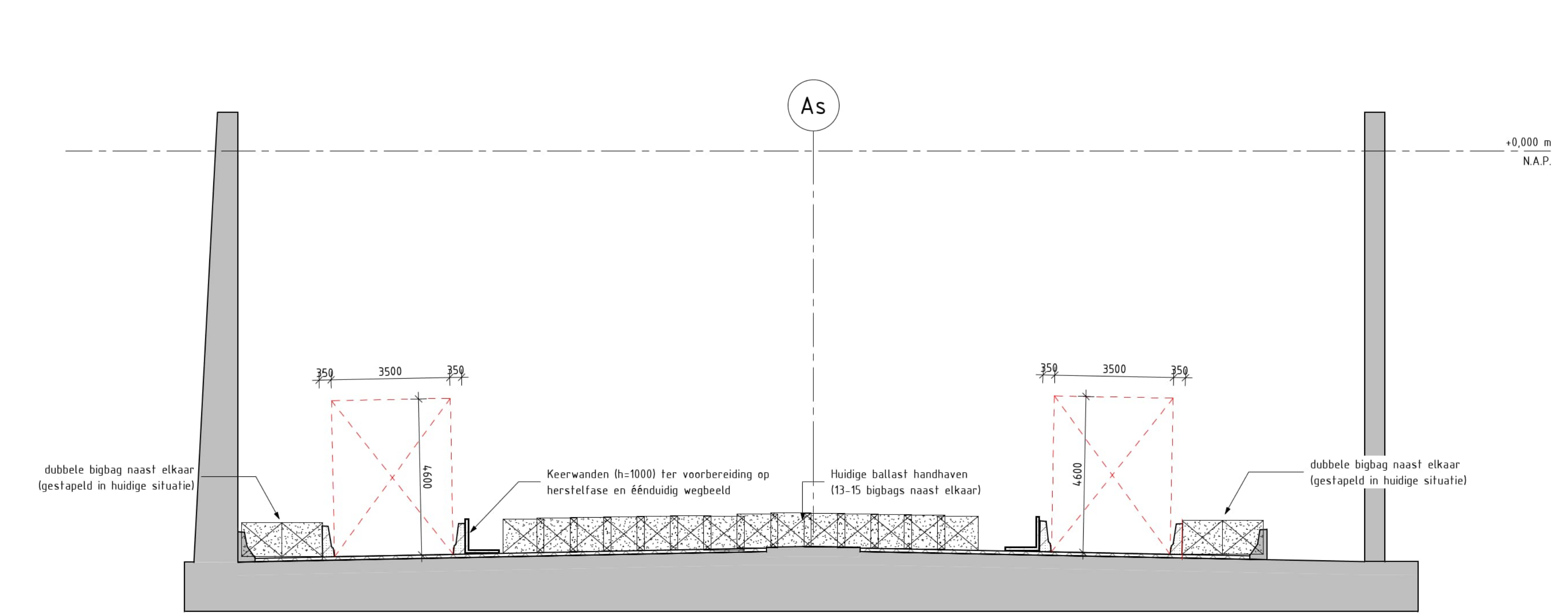
DOORSNEDE A-A (MOOT 20) schaal: 1:100
