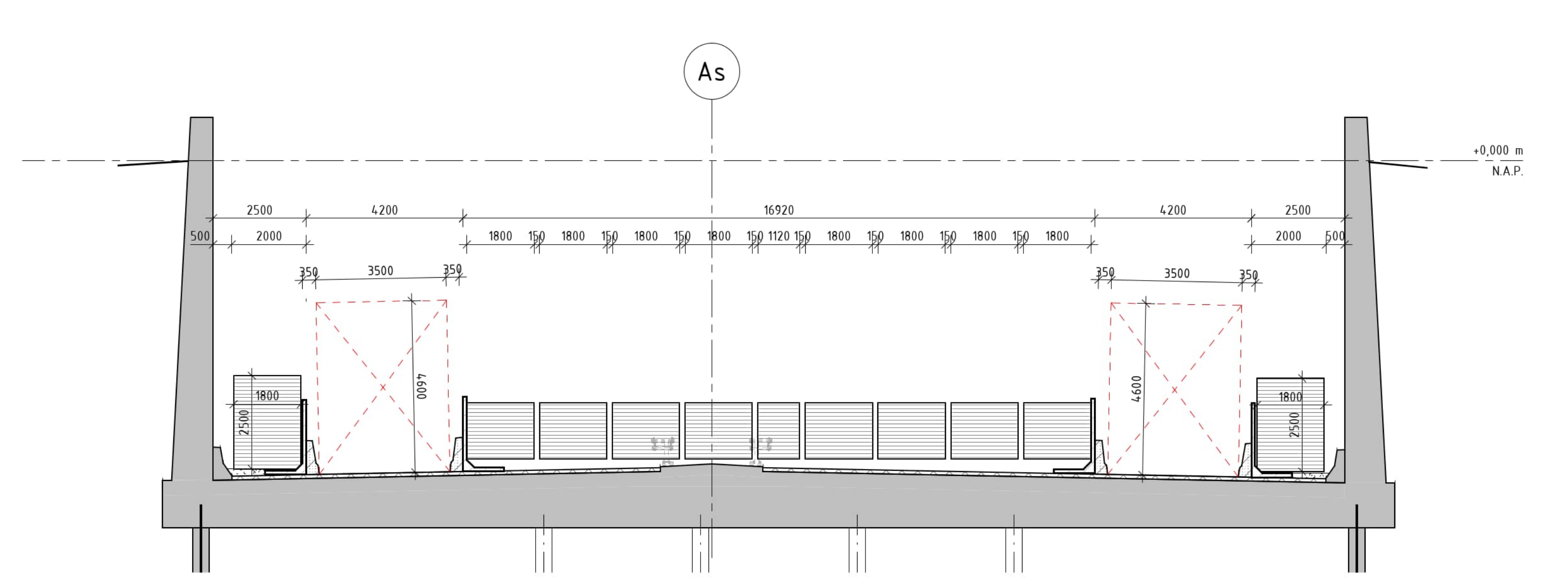
DOORSNEDE C-C (MOOT 26) schaal: 1:100
