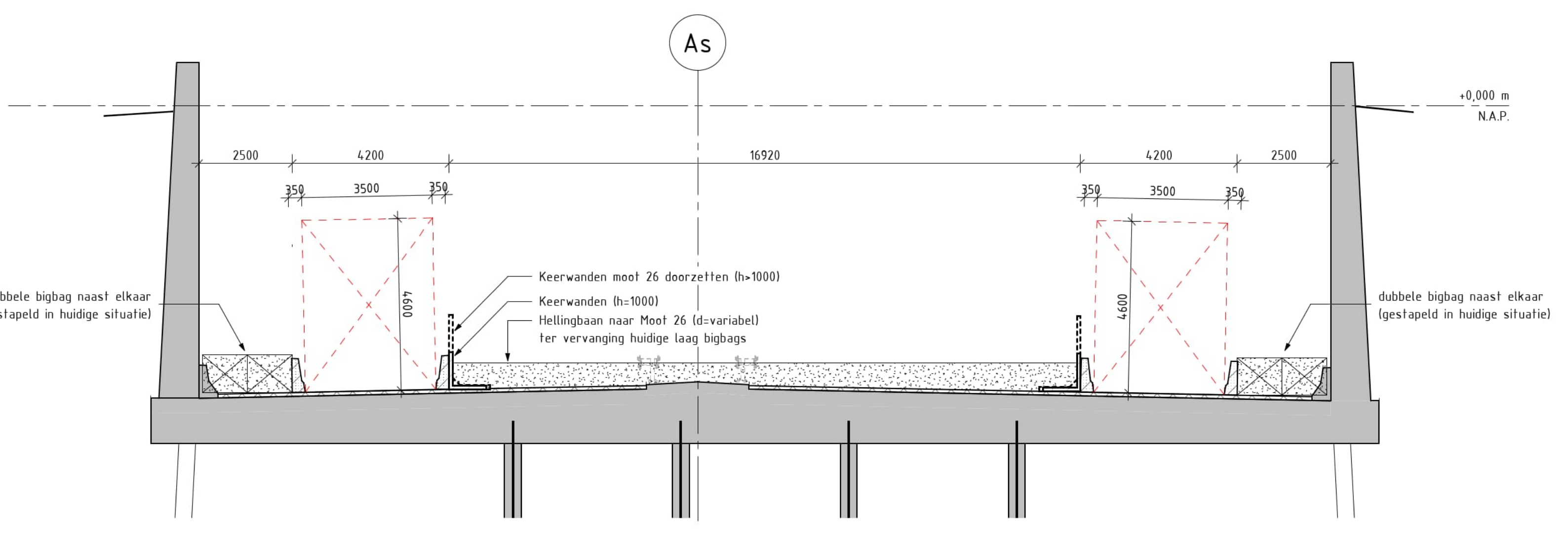
DOORSNEDE B-B (MOOT 27) schaal: 1:100
