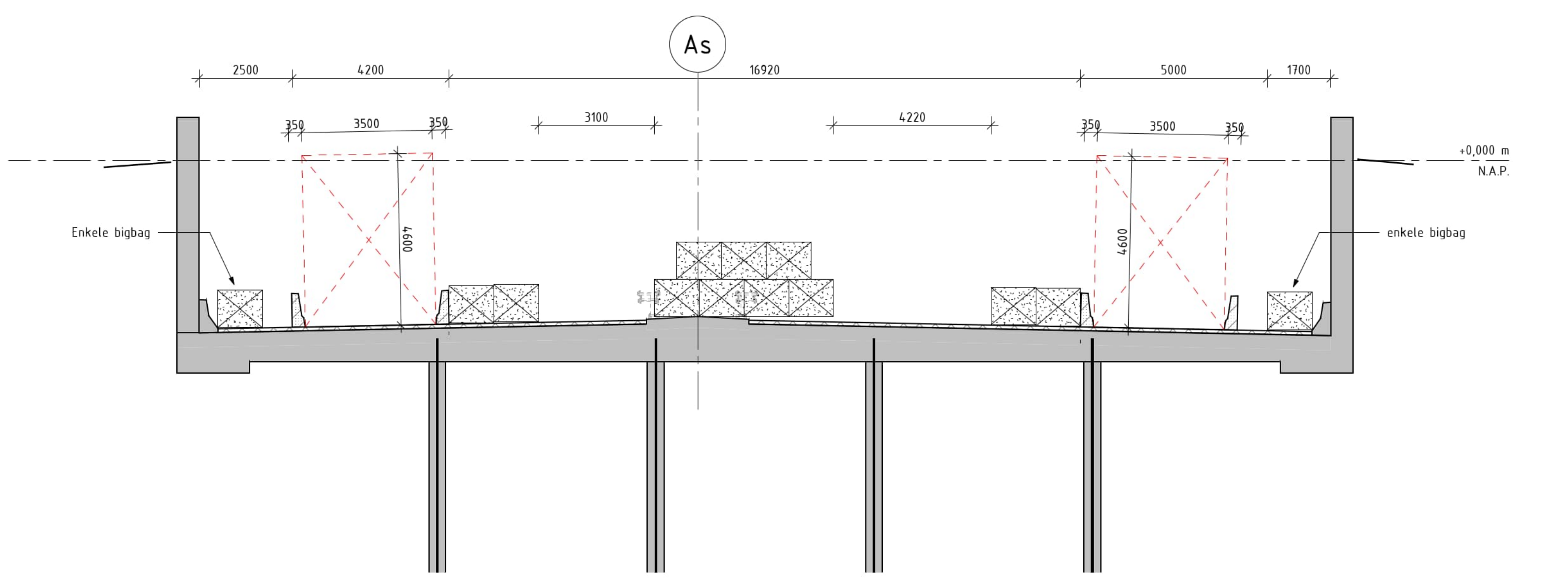
DOORSNEDE A-A (MOOT 32) schaal: 1:100
