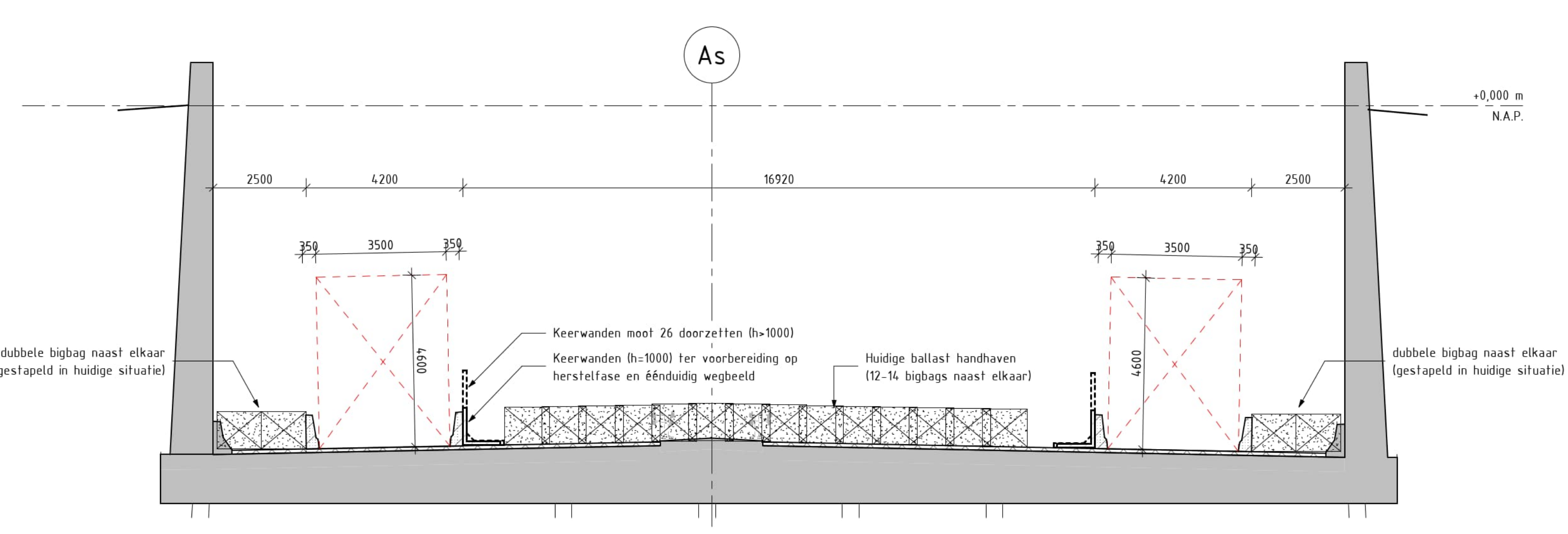
DOORSNEDE D-D (MOOT 25) schaal: 1:100
