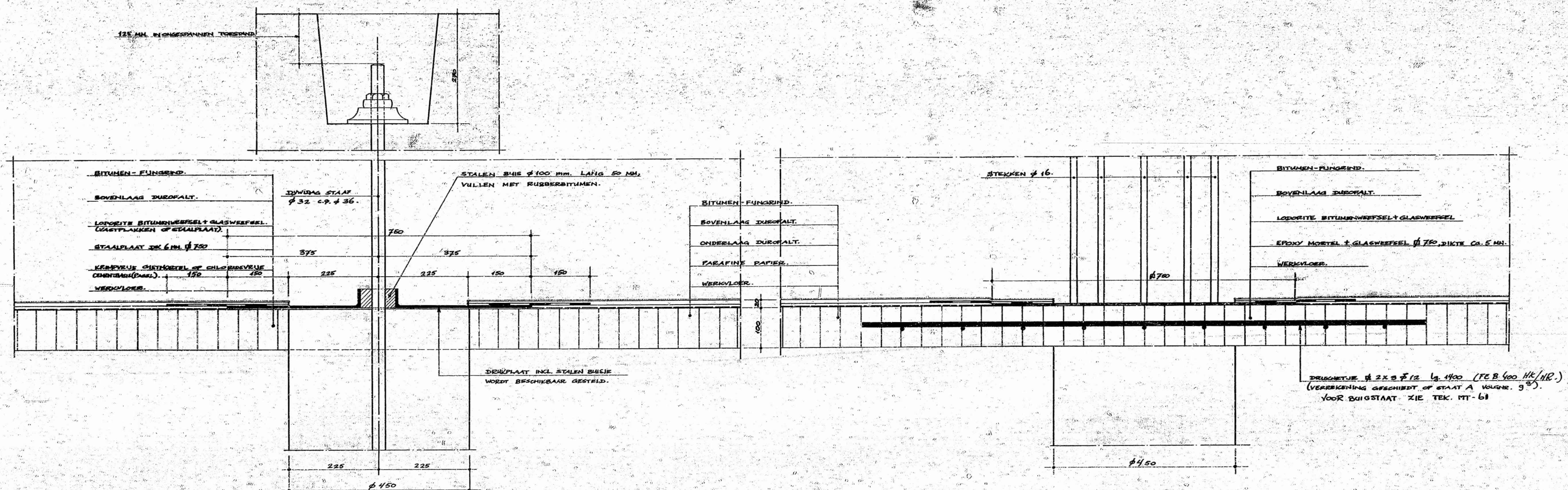
DETAIL TREKPAAL schaal: 1:5
