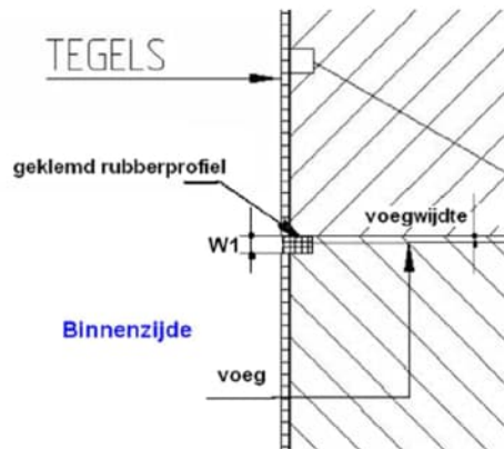
figuur D.6 Afwerking voeg aan binnenzijde met tegels
