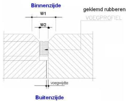
figuur D.5 Afwerking voeg aan binnenzijde zonder tegels.
