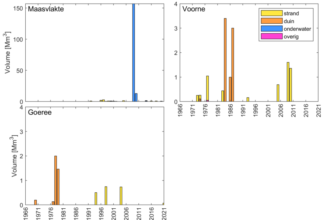
Figuur 3-4. Suppletievolumes tussen 1966 en april 2023 in de kustvakken bij de Haringvlietmondning (Goeree [12] vanaf raai 1225, Voorne [11] en Maasvlakte [10]) per suppletietype: strandsuppletie, duinverzwaring, onderwatersuppletie en overig.
