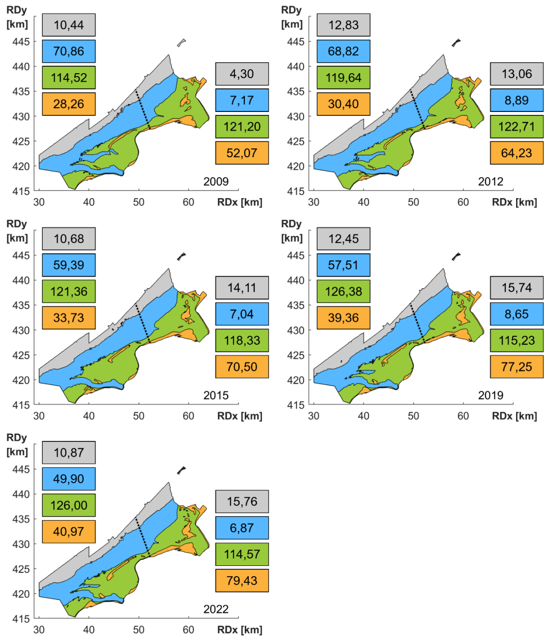
Figuur B 4. Overzicht van de absolute volumes [ Mm^3 ] binnen de diepe vooroever (grijs), de vooroever (blauw) de buitendelta (bestaande uit het platform (groen) en de banken (oranje)) voor de Grevelingen- en Haringvlietmonding voor 2009 t/m 2022.
