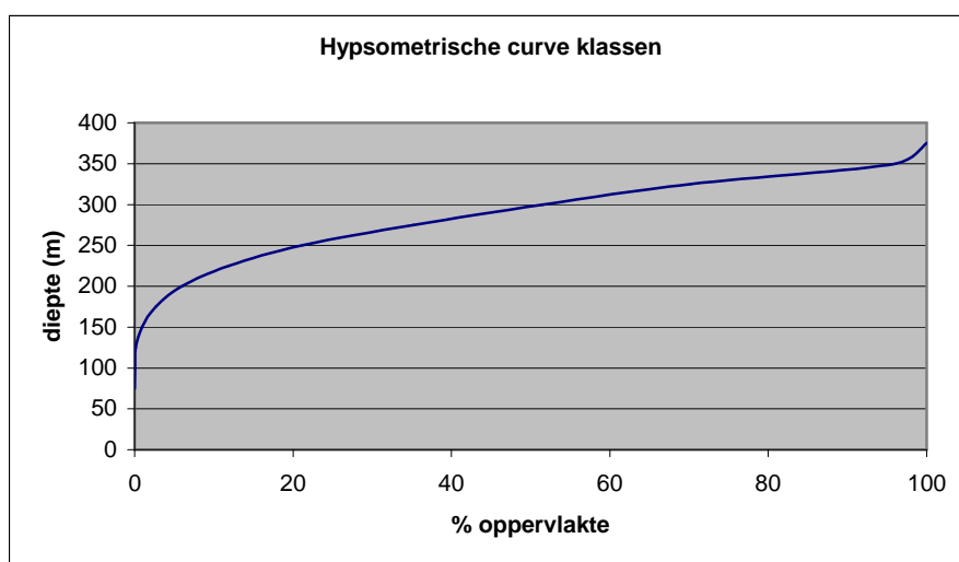
Figuur 4.8 Voorbeeld hypsometrische curve.
