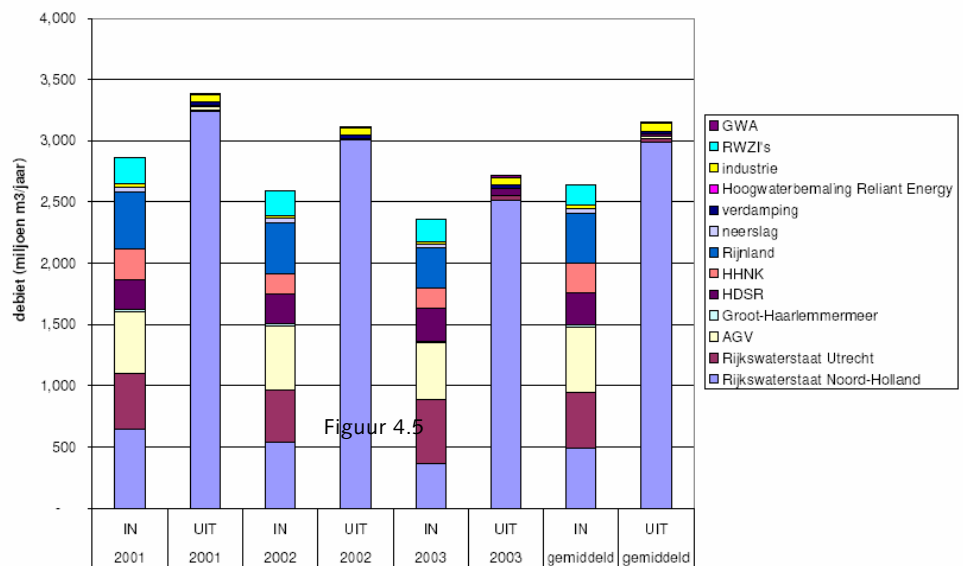
Figuur 4.5 Verdeling in- en uitdebiet op jaarbasis in miljoen m 3 /jaar voor Amsterdam-Rijnkanaal en Noordzeekanaal. (bron: waterbalans Noordzeekanaal/Amsterdam-Rijnkanaal 2001-2003, RWS Noord-Holland, 2005)
