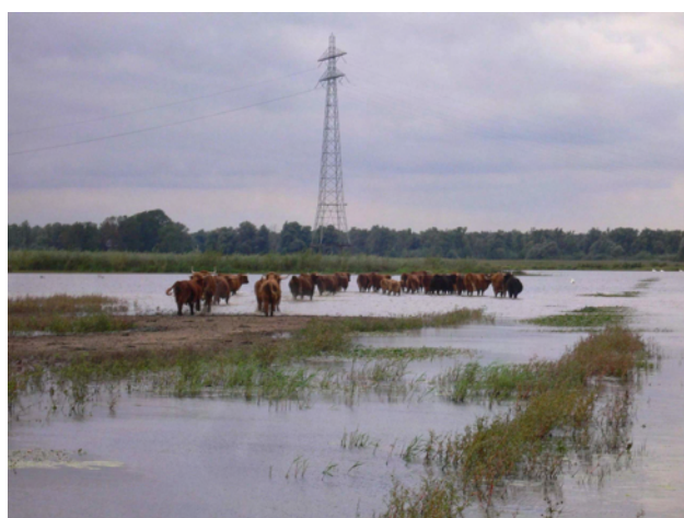
Figuur 3.27 en 3.28 Voorbeelden van inundatie (foto links: Waterschap Hollandse Delta; foto rechts: Ing. BCC)
