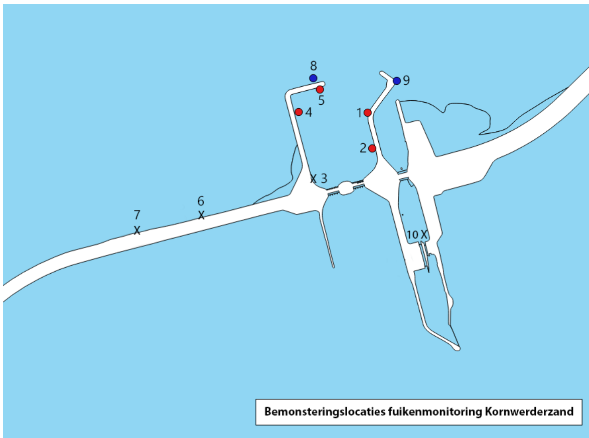
Figuur 6.7 Overzicht van de fuiklocaties in en buiten de spuikom bij Kornwerderzand. Fuiken 1-7 zijn van het reguliere programma, fuiken 8-10 zijn de additionele fuiken waarmee gevist is in 2013 en 2014. In 2022 zijn fuiken 3, 6 en 7 wegens werkzaamheden komen te vervallen en zijn fuik 8 en 9 opgenomen in het bemonsteringsprogramma.
