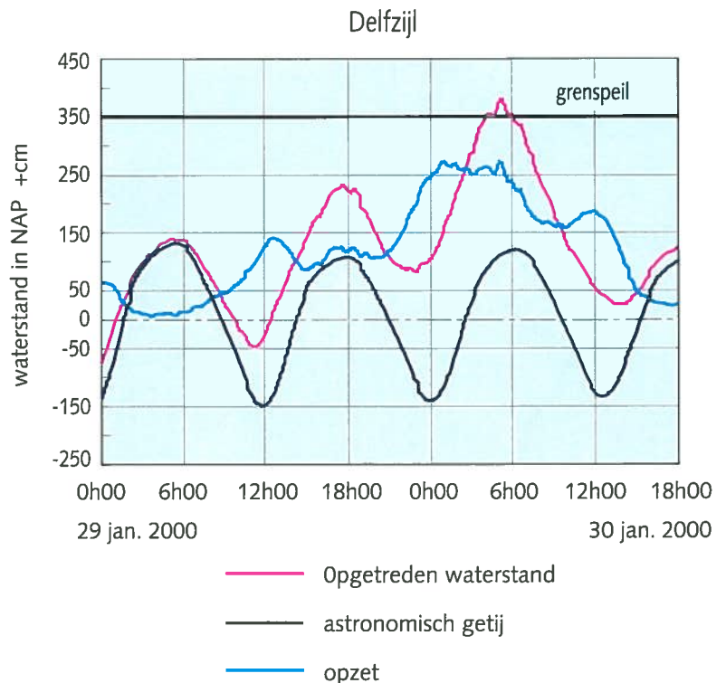
Figuur 5 Waterstandsverloop van Delfzijl
