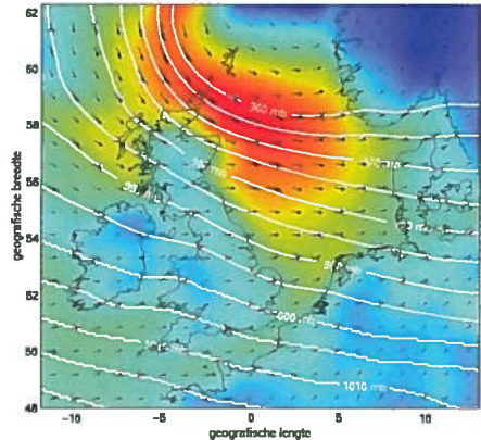
Wind en druk, KNMI voorspelling voor 29-Jan-2000 18:00:00 GMT, (3 uur na analyse)
