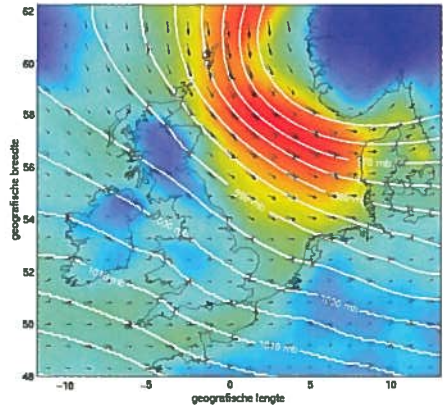
Wind en druk, KNMI voorspelling voor 29-Jan-2000 21:00:00 GMT, (9 uur na analyse)
