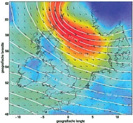
Wind en druk, KNMI voorspelling voor 29-Jan-2000 18:00:00 GMT, (6 uur na analyse)
