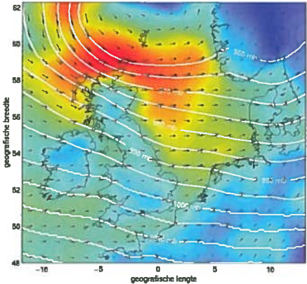
Wind en druk, KNMI voorspelling voor 29-Jan-2000 12:00:00 GMT, (0 uur na analyse)
