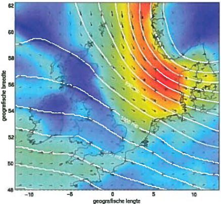
Wind en druk, KNMI voorspelling voor 30-Jan-2000 00:00:00 GMT, (0 uur na analyse)
