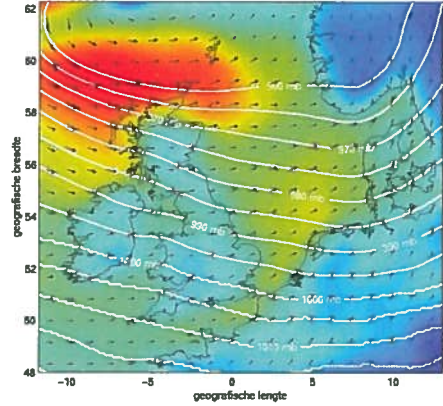
Wind en druk, KNMI voorspelling voor 29-Jan-2000 09:00:00 GMT, (3 uur na analyse)
