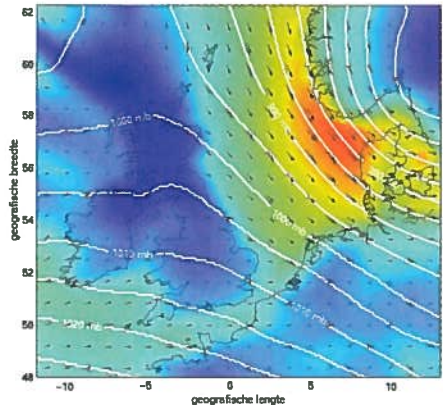
Wind en druk, KNMI voorspelling voor 30-Jan-2000 03:00:00 GMT, (3 uur na analyse)
