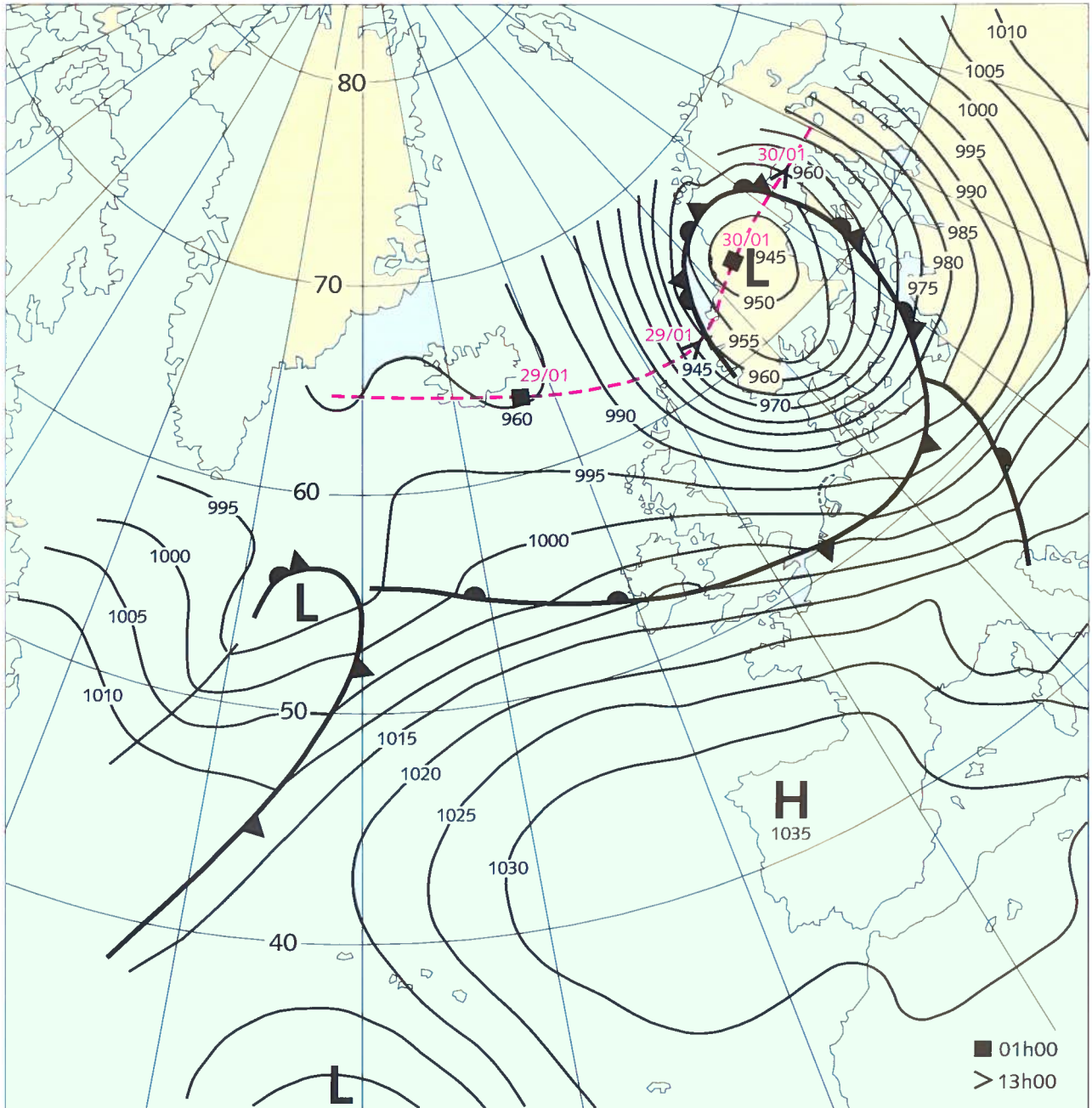
Depressiebaan en luchtdrukverdeling van 30 januari 01h00.
