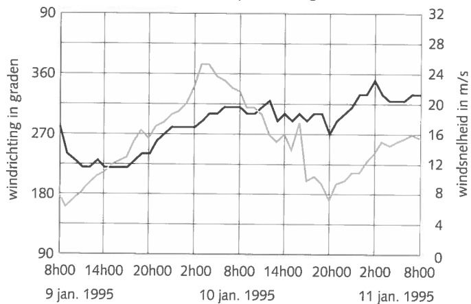
Windverloop Huibergat
