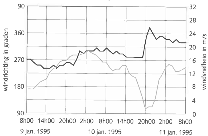
Windverloop IJmuiden
