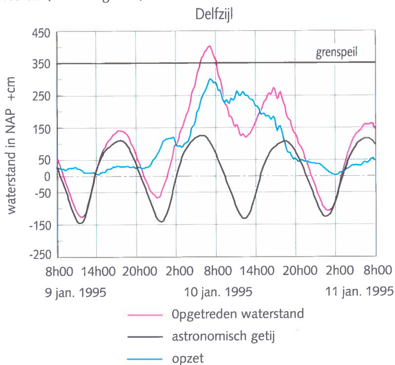
Figuur 4 Waterstandsverloop Delfzijl
