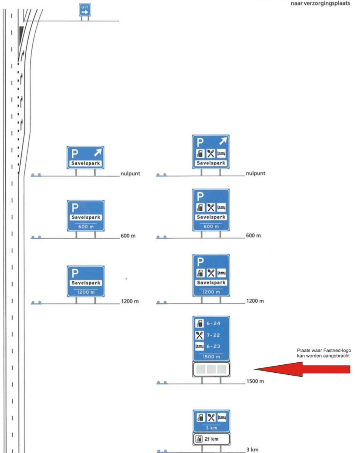
Figuur 3.31. Enkelstrooksuitvoeging naar verzorgingsplaats
