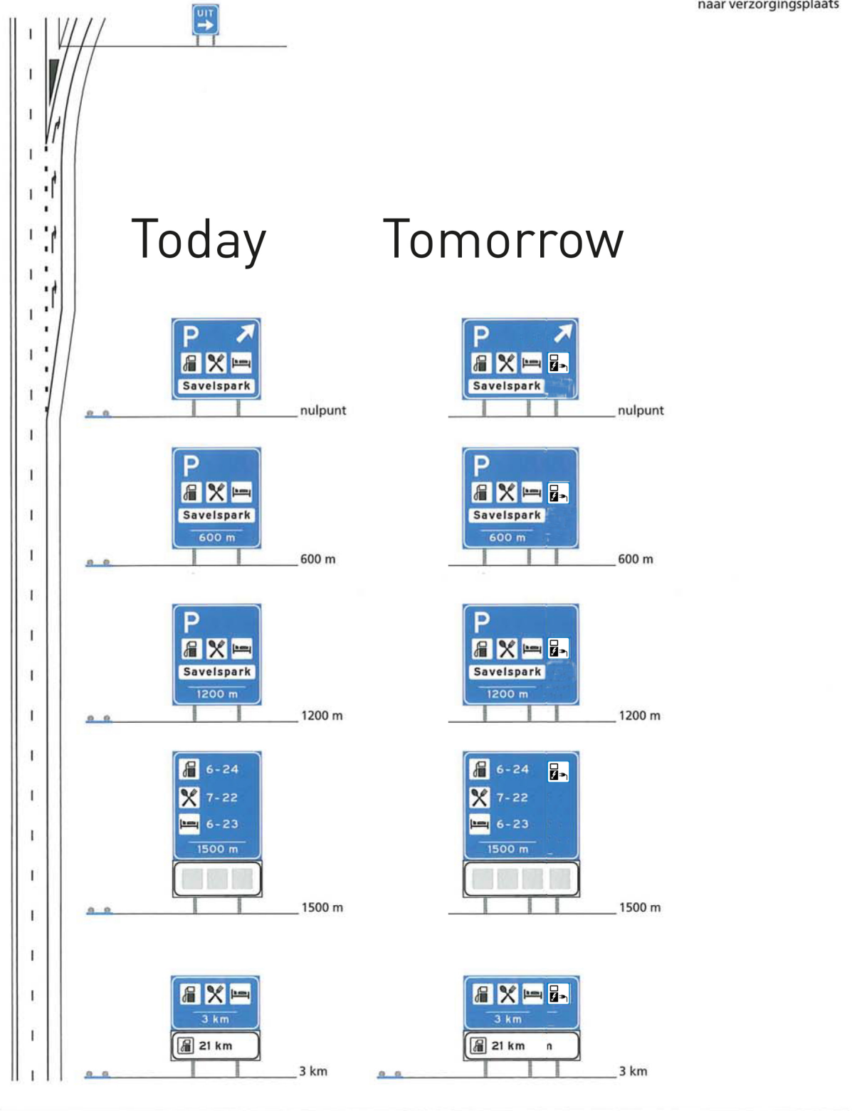
Figuur 3.31. Enkelstrooksuitvoeging naar verzorgingsplaats
