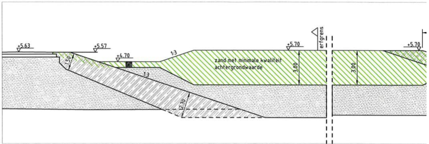
Doorsnede A
