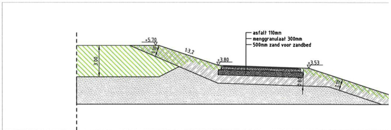
Doorsnede B
