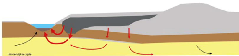
Schematische weergave van het dijklichaam met hierin met pijlen de grondwaterstroming (rode én zwarte pijlen) en beweging van uit de TGG gemobiliseerde (vervuilende) stoffen (met rode pijlen). De grootste effecten bevinden zich in de veenlaag die direct in contact staat met de TGG en in de aangrenzende teensloot (dikke pijlen).
