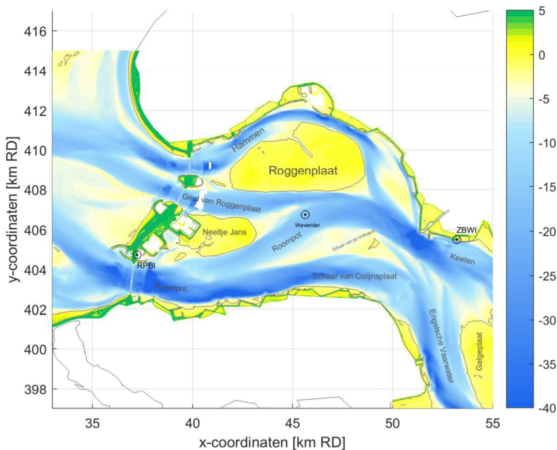
Figuur 2.2 Bodemligging Roggenplaat en omgeving (2013) met de belangrijkste geulen en platen. Ook de locatie van de Waverider en de meetstations Roompot Binnen (waterstanden) en Zeelandbrug Wind zijn weergegeven.
