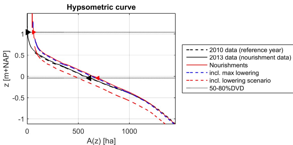
Figuur 5.4 Uitwerking zandbron suppletievariant.
