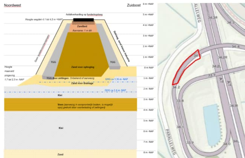
Figuur 6.2 Dwarsdoorsnede en ligging conceptueel model A7 Hoom Afrit 9
