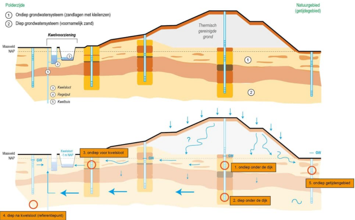
Figuur 7: Schematische weergave van de grondwatermonitoringspunten.
