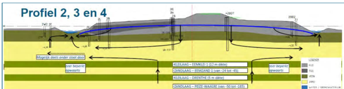
Figuur 2.3: Principeschets gedrag grondwater
