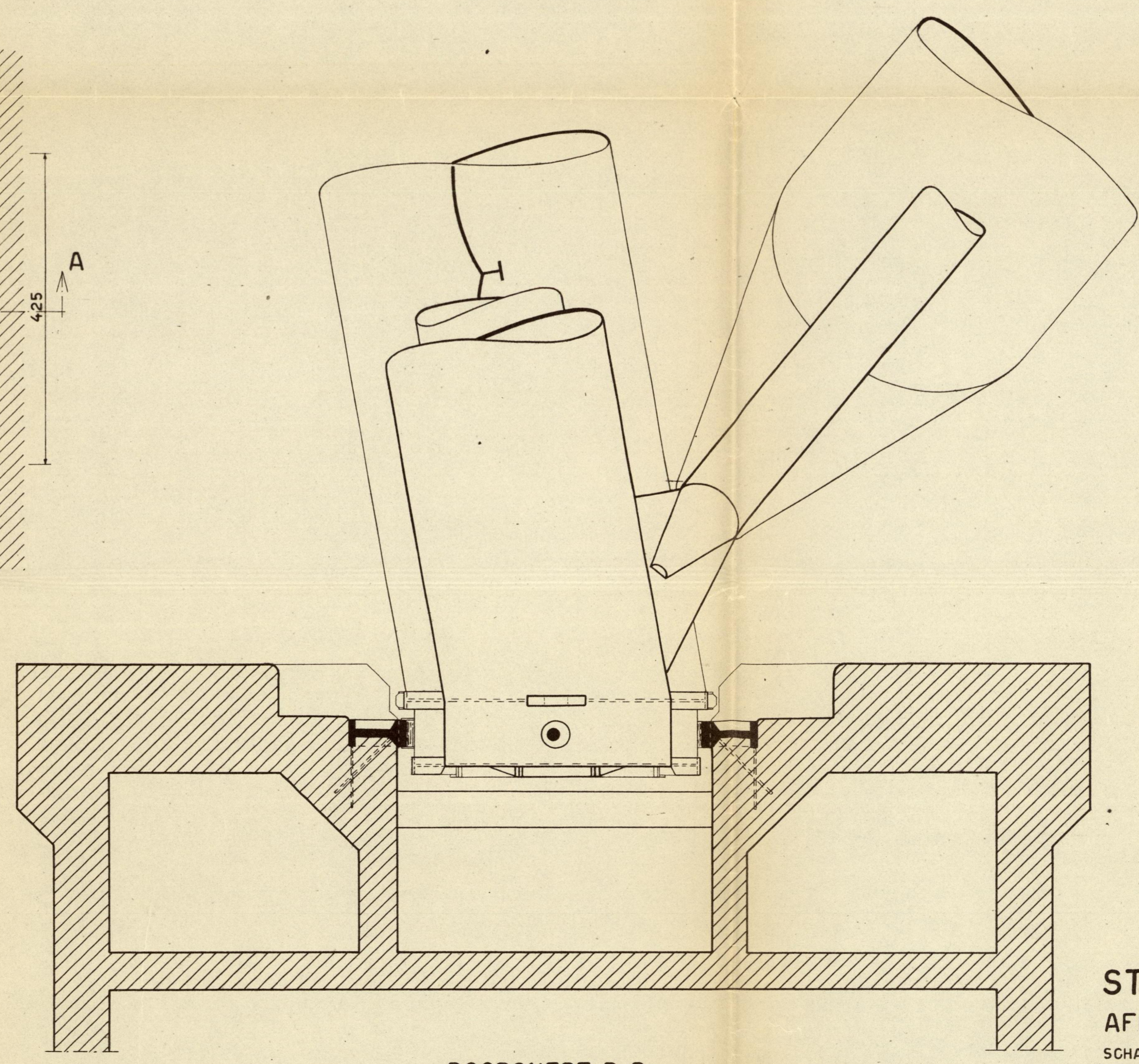
DOORSNEDE D-D
