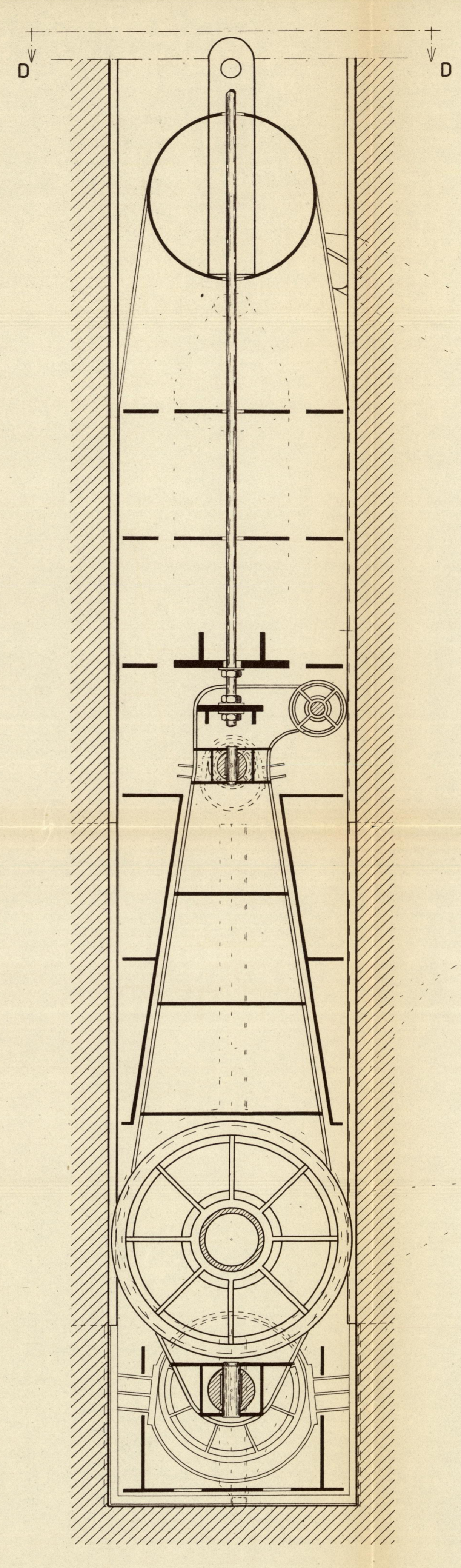
DOORSNEDE B-B
