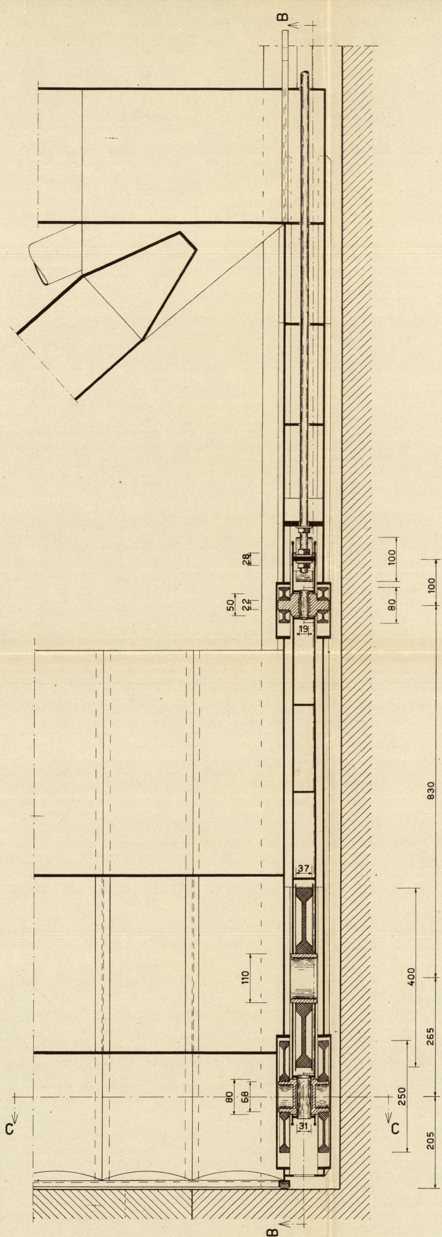
DOORSNEDE A-A
