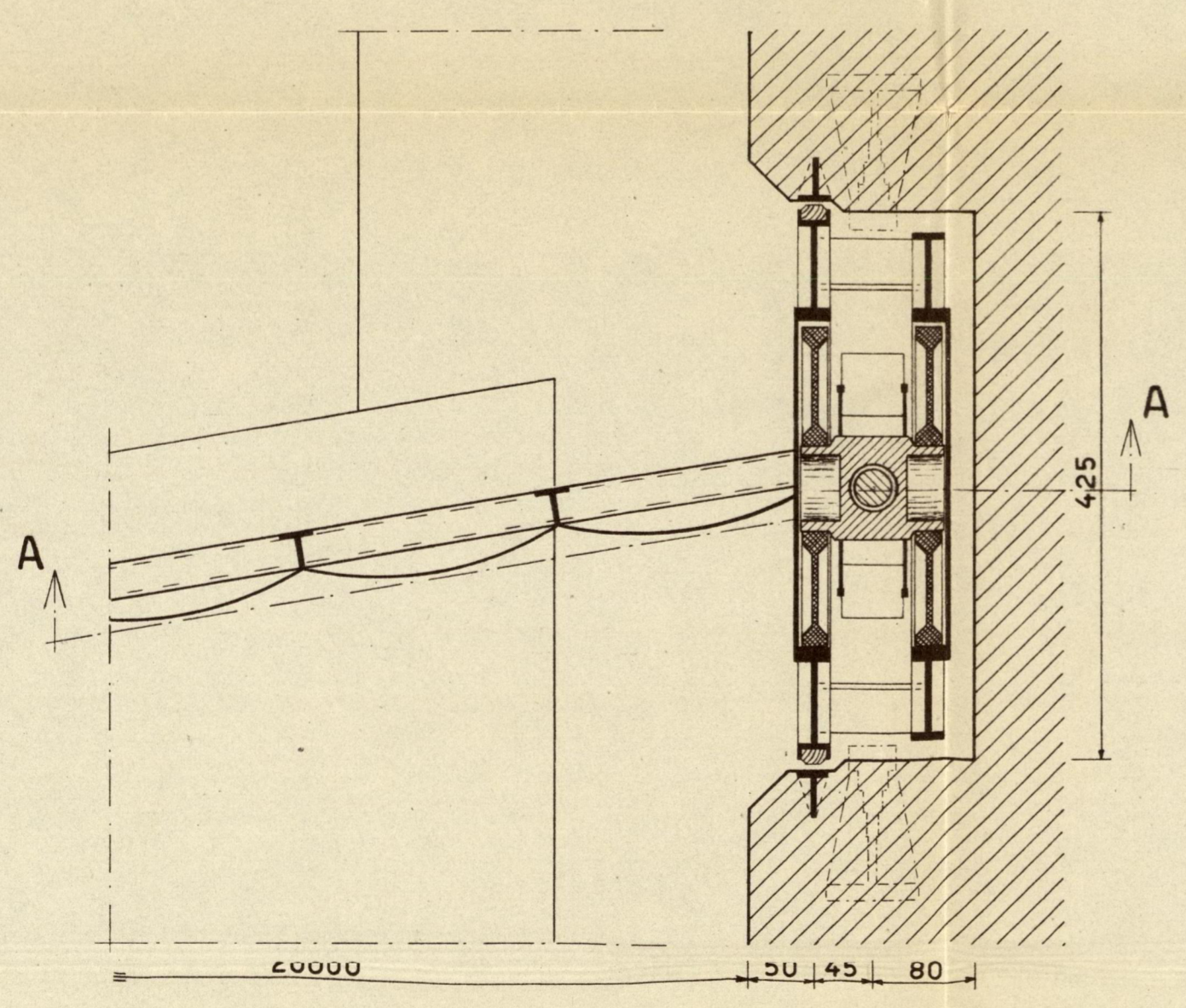
DOORSNEDE C-C
