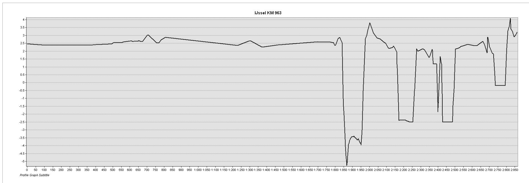
Afbeelding III.10 Dwarsprofiel huidige bodemligging IJssel (KM 963) uit Baseline
