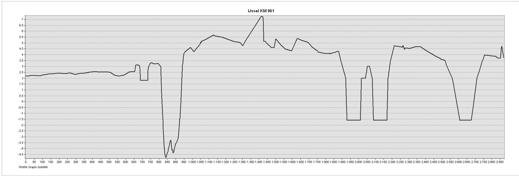
Afbeelding III.8 Dwarsprofiel huidige bodemligging IJssel (KM 955) uit Baseline
