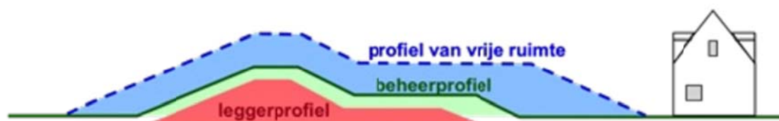
Figuur 2-7: Profiel van de vrije ruimte. Bron. www.stowa.nl .
