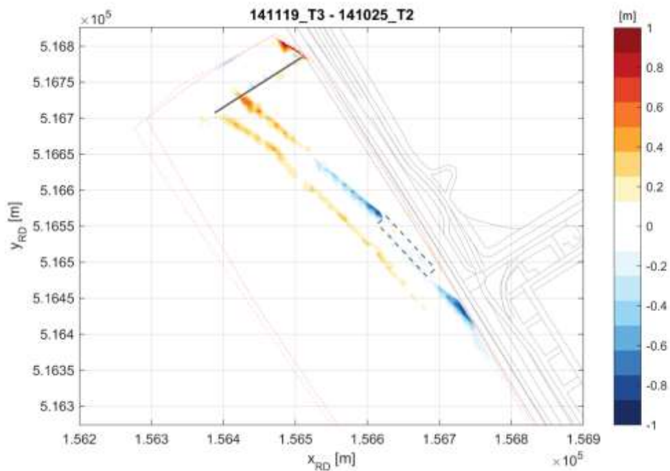
Figuur 6-24 Verschil in bodemligging tussen T2- en T3-opname.
