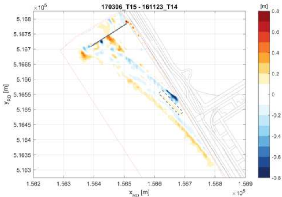
Figuur 6-36 Verschil in bodemligging tussen T14- en T15-opname.
