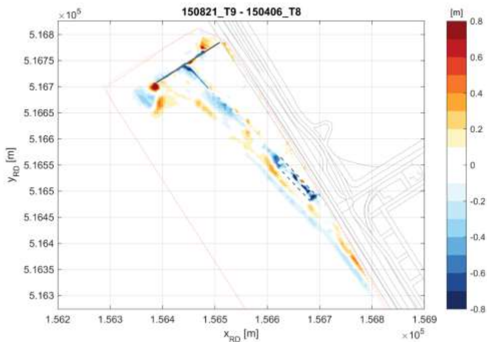
Figuur 6-30 Verschil in bodemligging tussen T8- en T9-opname.
