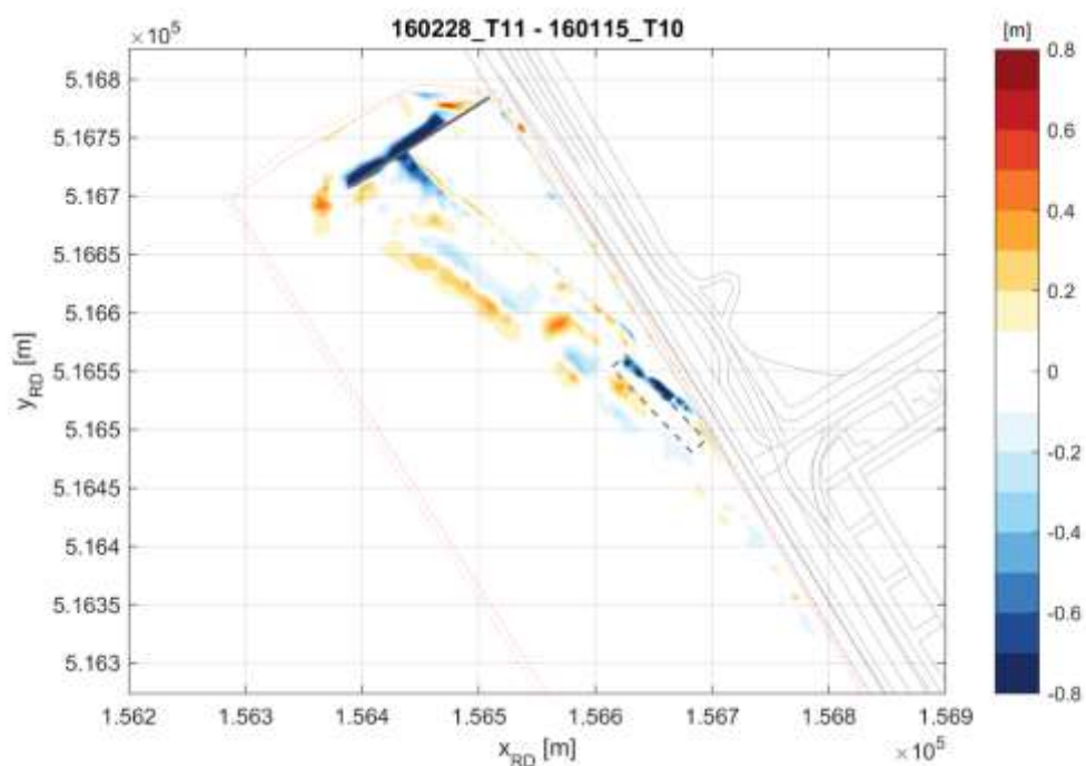
Figuur 6-32 Verschil in bodemligging tussen T10- en T11-opname.
