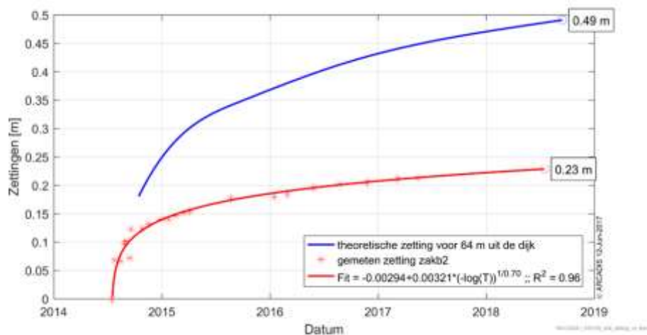
Figuur 6-59 Gemeten zettingen in zakb2 vergeleken met de theoretische zetting voor dit punt.
