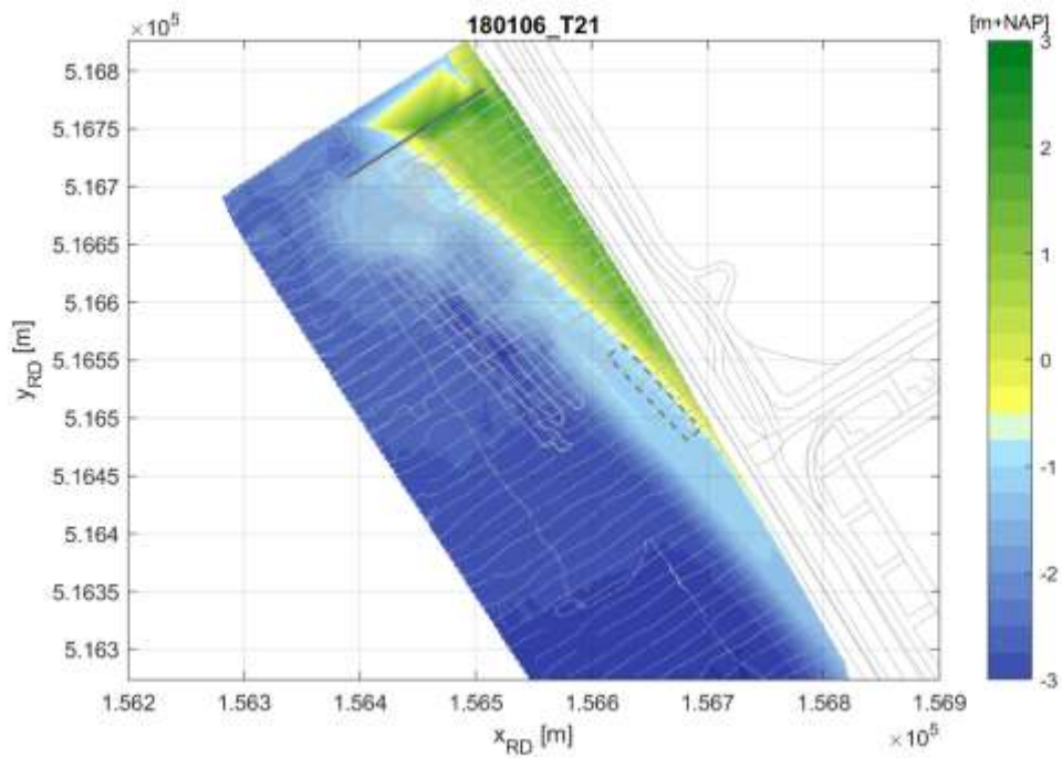
Figuur 6-22 Overzicht bodemligging T21-inmeting op 6 januari 2017.
