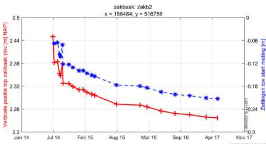
Figuur 6-42 Absolute ontwikkeling top van het zakbaken voor zakb2 (rode lijn), samen met de bijbehorende zetting (blauwe lijn).
