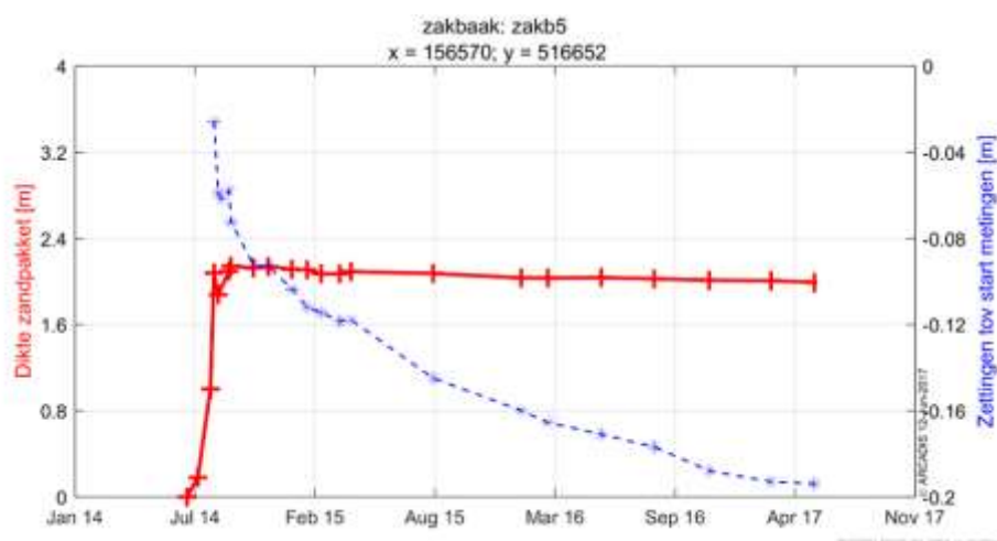
Figuur 6-52 Opgetreden zettingen in relatie met de dikte van het zandpakket in zakb5.
