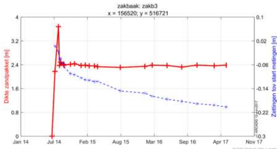
Figuur 6-50 Opgetreden zettingen in relatie met de dikte van het zandpakket in zakb3.
