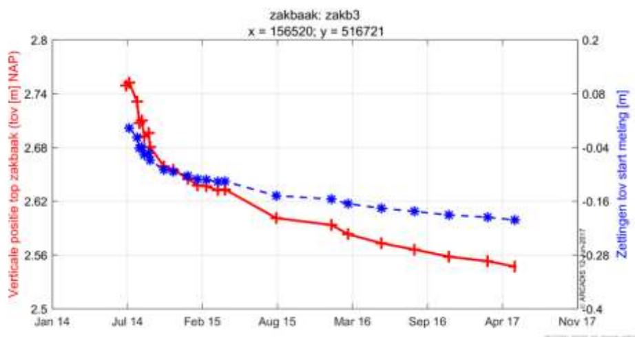
Figuur 6-43 Absolute ontwikkeling top van het zakbaken voor zakb3 (rode lijn), samen met de bijbehorende zetting (blauwe lijn).
