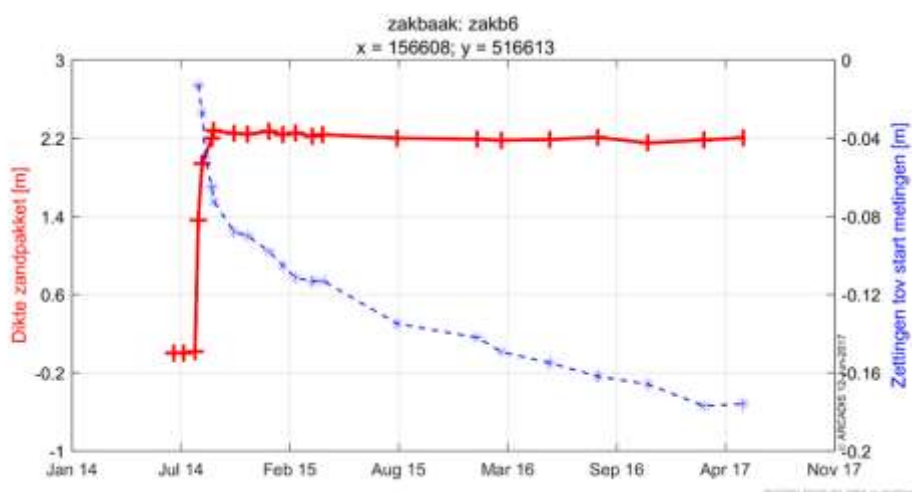
Figuur 6-53 Opgetreden zettingen in relatie met de dikte van het zandpakket in zakb6.
