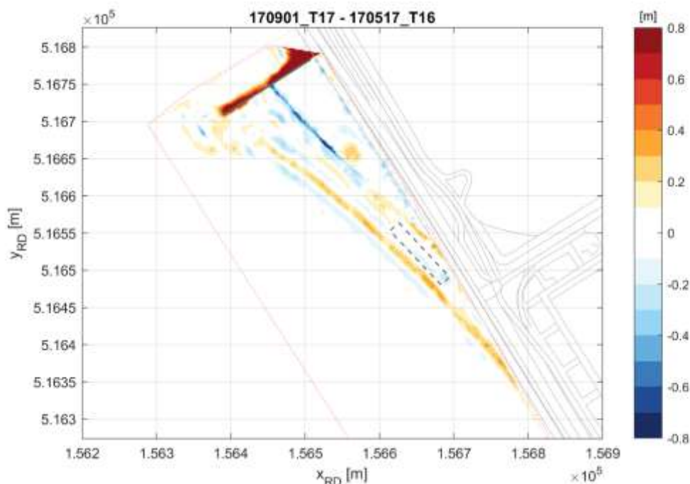
Figuur 6-38 .....Verskil in bodemligging tussen T16- en T17-opname. ..... 124
