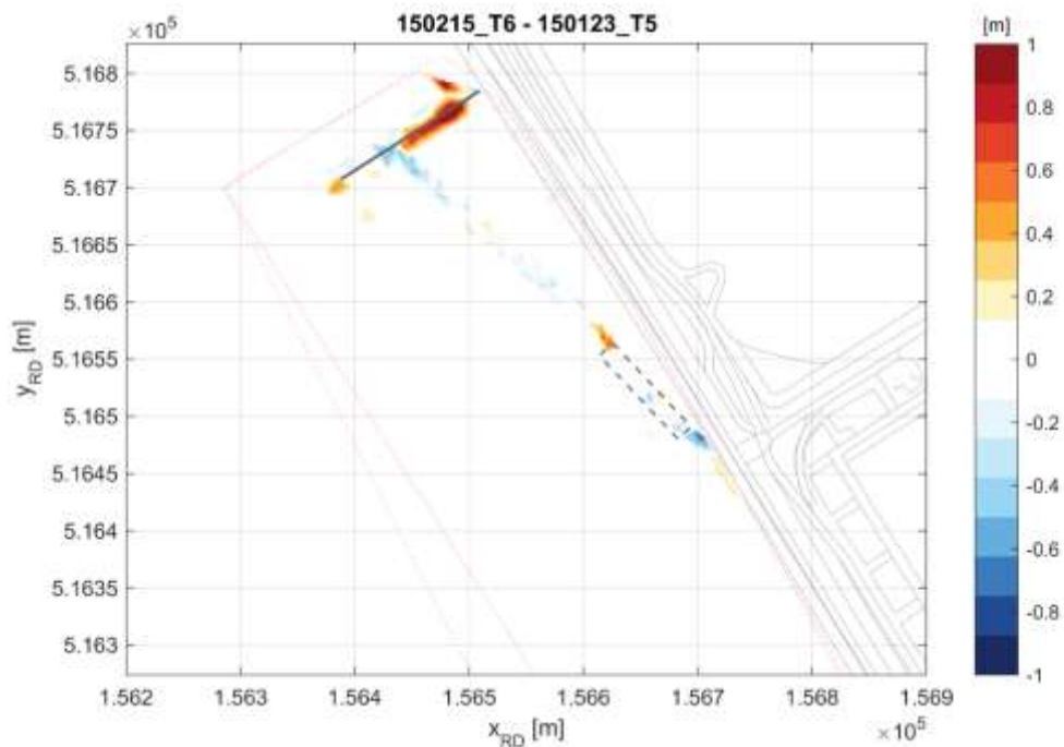
Figuur 6-27 Verschil in bodemligging tussen T5- en T6-opname.
