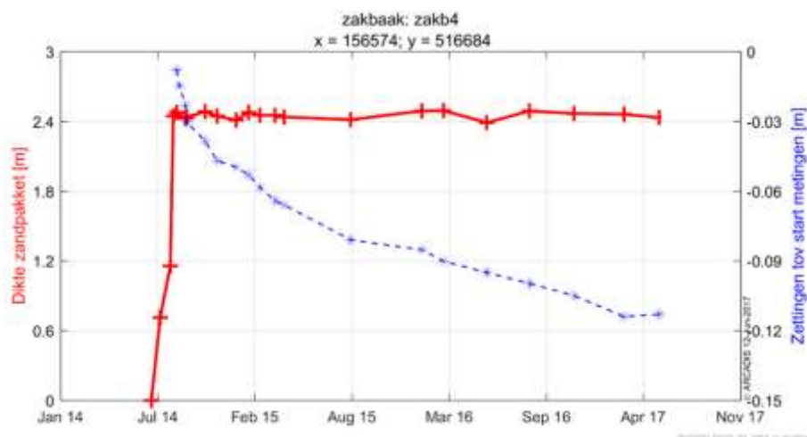
Figuur 6-51 Opgetreden zettingen in relatie met de dikte van het zandpakket in zakb4.
