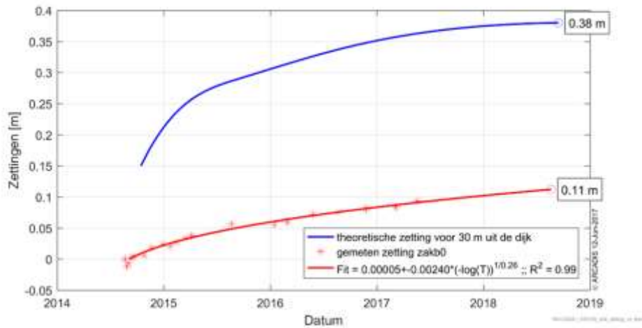
Figuur 6-57 Gemeten zettingen in zakb0 vergeleken met de theoretische zetting voor dit punt.
