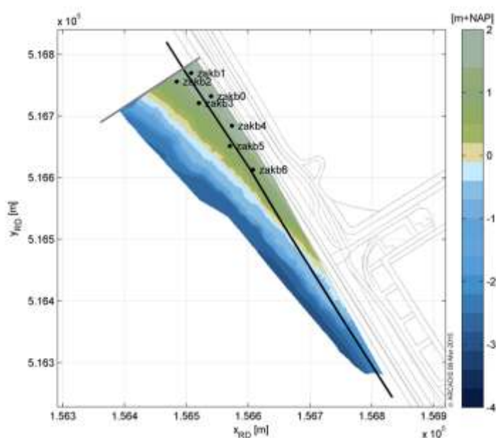
Figuur 6-39 Overzicht positie van de zeven geplaatste zakbakens, inclusief de veronderstelde positie van de buitenbegrenzing van het cunet (zwarte lijn).
