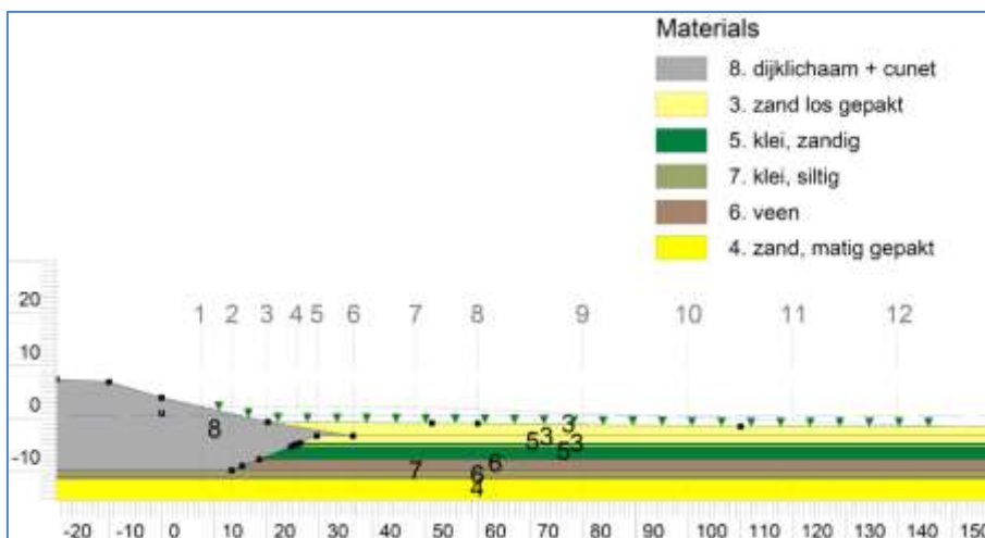
Figuur 6-54 Schematisatie ondergrond Houtribdijk ter plaatse van pilot.
