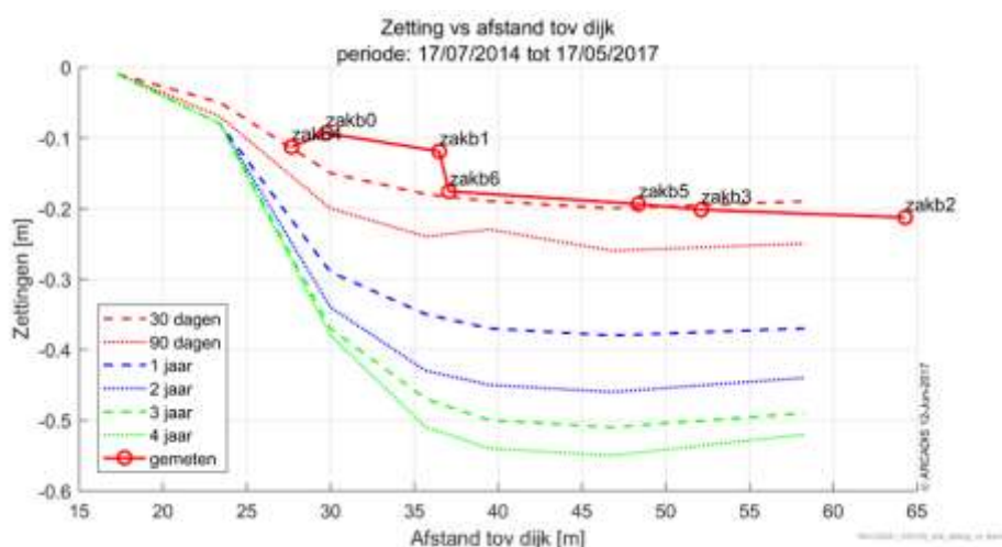
Figuur 6-56 Gemeten zettingen in kustwaarsrichting vergeleken met de voorspelde zettingen op meerdere momenten in de tijd.
