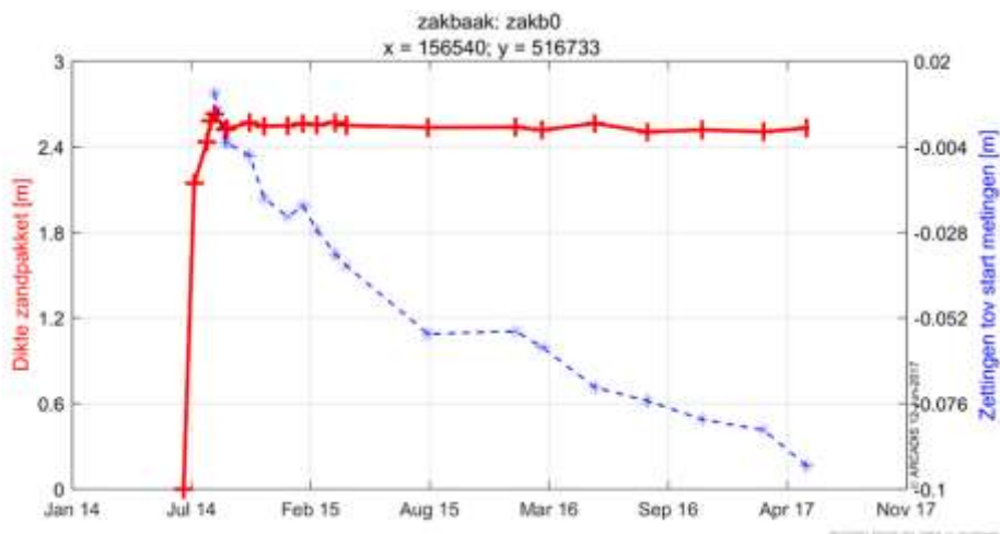
Figuur 6-47 Opgetreden zettingen in relatie met de dikte van het zandpakket in zakb0.
