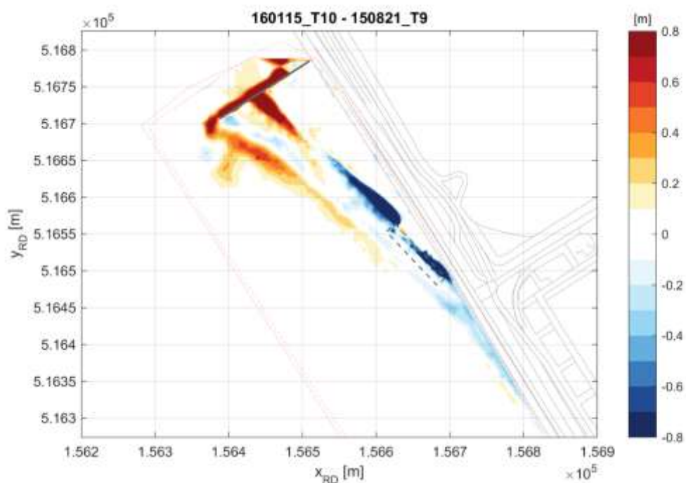
Figuur 6-31 Verschil in bodemligging tussen T9- en T10-opname.
