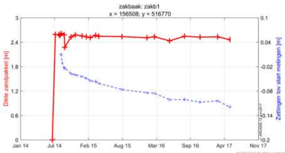
Figuur 6-48 Opgetreden zettingen in relatie met de dikte van het zandpakket in zakb1.
