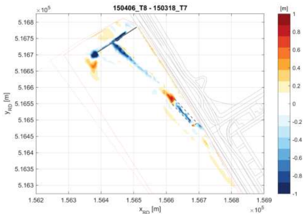
Figuur 6-29 Verschil in bodemligging tussen T7- en T8-opname.
