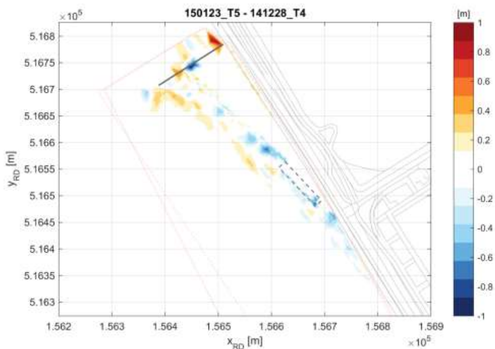
Figuur 6-26 Verschil in bodemligging tussen T4- en T5-opname.
