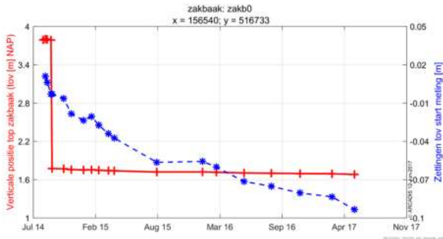
Figuur 6-40 Absolute ontwikkeling top van het zakbaken voor zakb0 (rode lijn), samen met de bijbehorende zetting (blauwe lijn).
