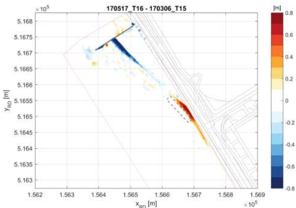
Figuur 6-37 Verschil in bodemligging tussen T15- en T16-opname.
