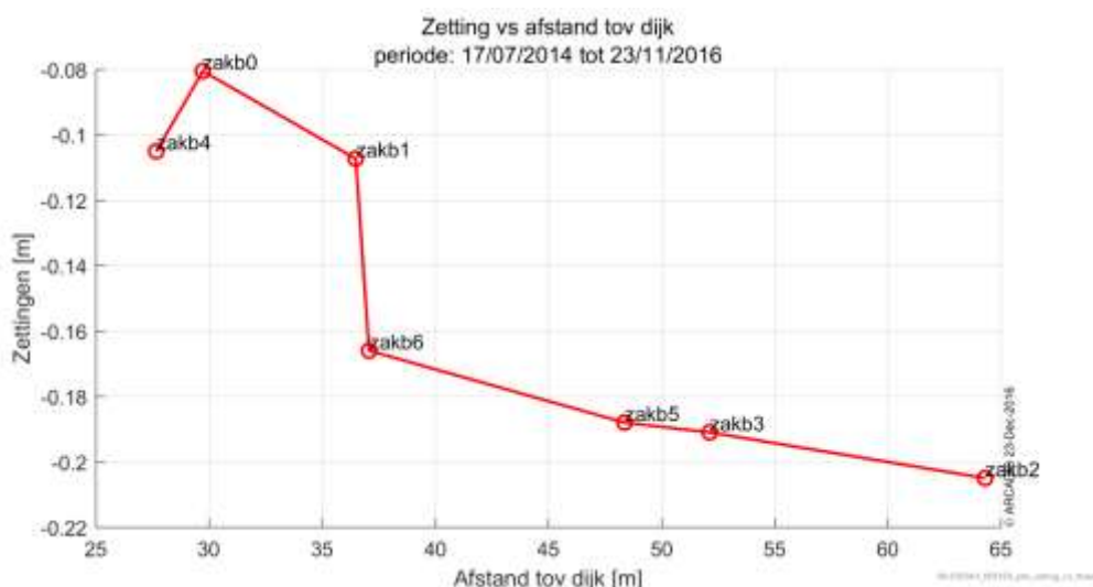
Figuur 6-55 Gemeten zettingen uitgezet tegen de afstand in kustwaarsrichting.
