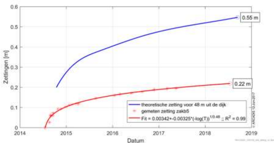
Figuur 6-62 Gemeten zettingen in zakb5 vergeleken met de theoretische zetting voor dit punt.
