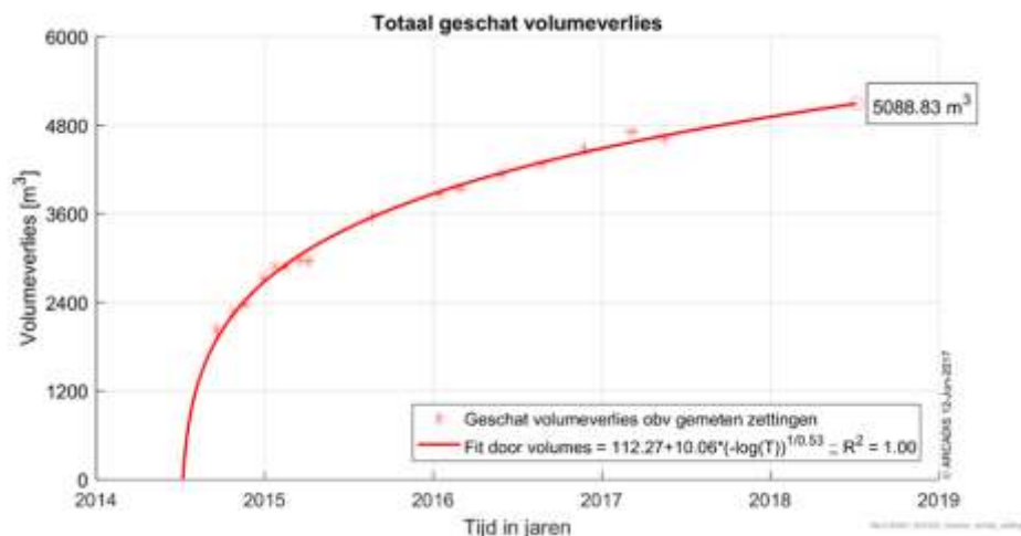
Figuur 6-64 Geschat verloop van het zetting gerelateerd volumeverlies.
