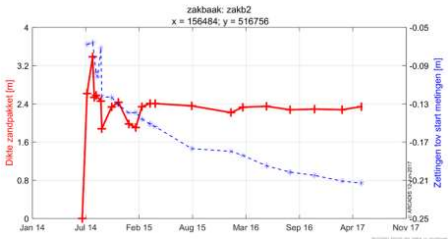
Figuur 6-49 Opgetreden zettingen in relatie met de dikte van het zandpakket in zakb2.
