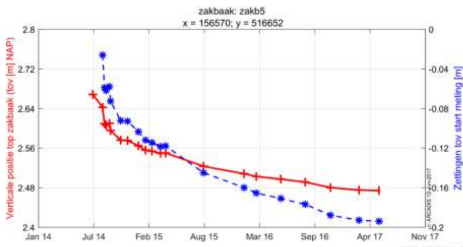
Figuur 6-45 Absolute ontwikkeling top van het zakbaken voor zakb5 (rode lijn), samen met de bijbehorende zetting (blauwe lijn).
