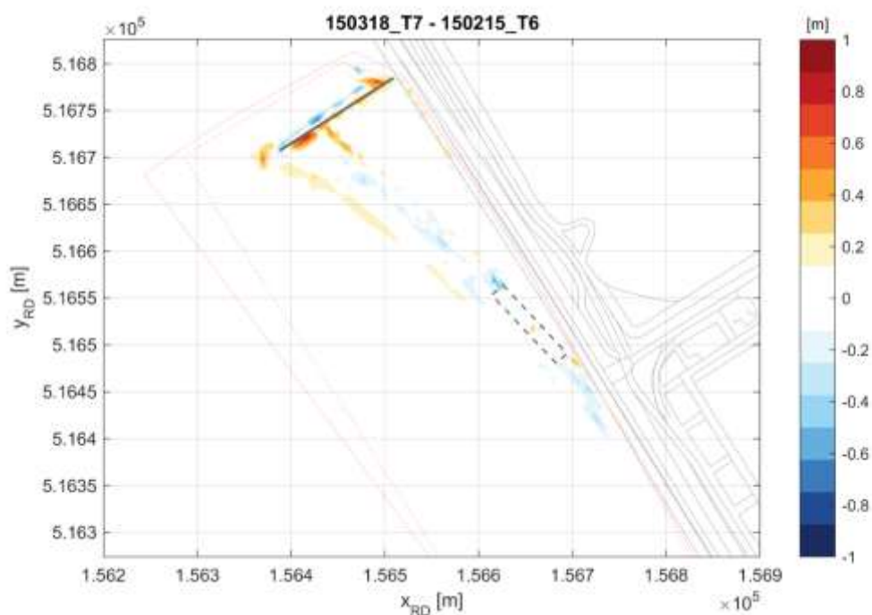
Figuur 6-28 Verschil in bodemligging tussen T6- en T7-opname.
