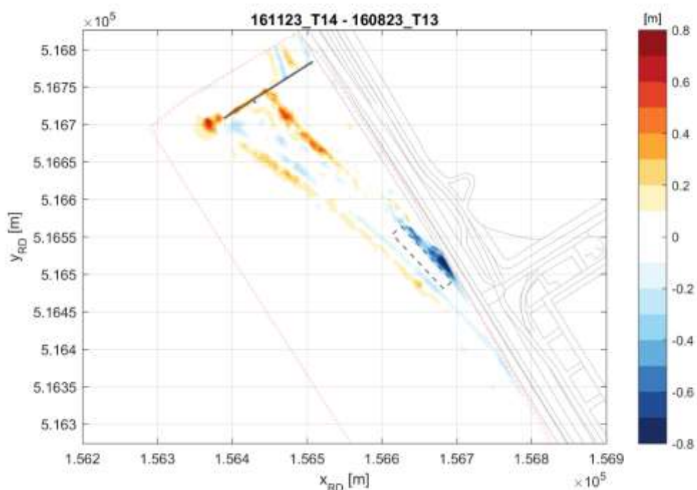
Figuur 6-35 Verschil in bodemligging tussen T13- en T14-opname.
