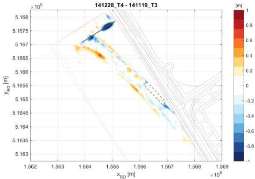
Figuur 6-25 Verschil in bodemligging tussen T3- en T4-opname.
