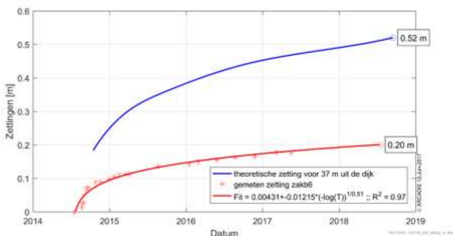
Figuur 6-63 Gemeten zettingen in zakk6 vergeleken met de theoretische zetting voor dit punt.
