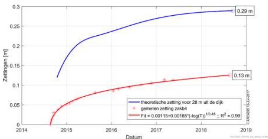
Figuur 6-61 Gemeten zettingen in zakb4 vergeleken met de theoretische zetting voor dit punt.
