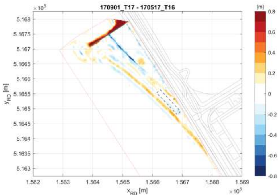
Figuur 6-38 Verschil in bodemligging tussen T16- en T17-opname.
