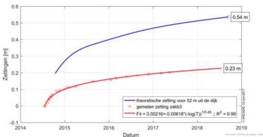
Figuur 6-60 Gemeten zettingen in zakb3 vergeleken met de theoretische zetting voor dit punt.
