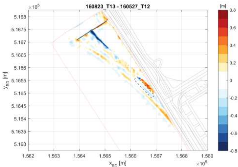
Figuur 6-34 Verschil in bodemligging tussen T12- en T13-opname.
