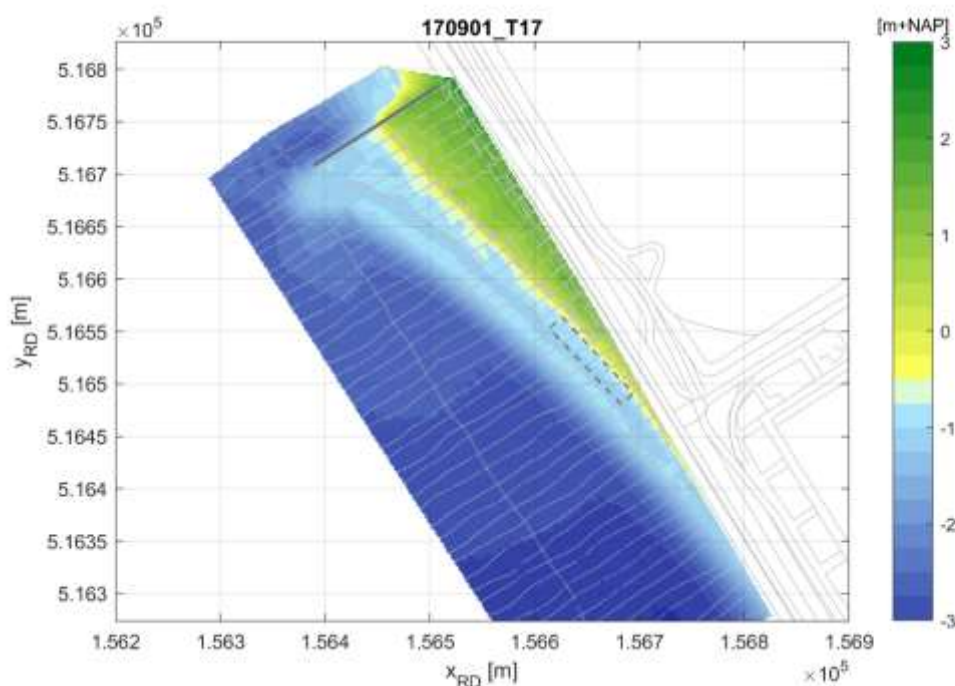
Figuur 6-18 Overzicht bodemligging T17-inmeting op 1 september 2017 (laatste reguliere inmeting).
