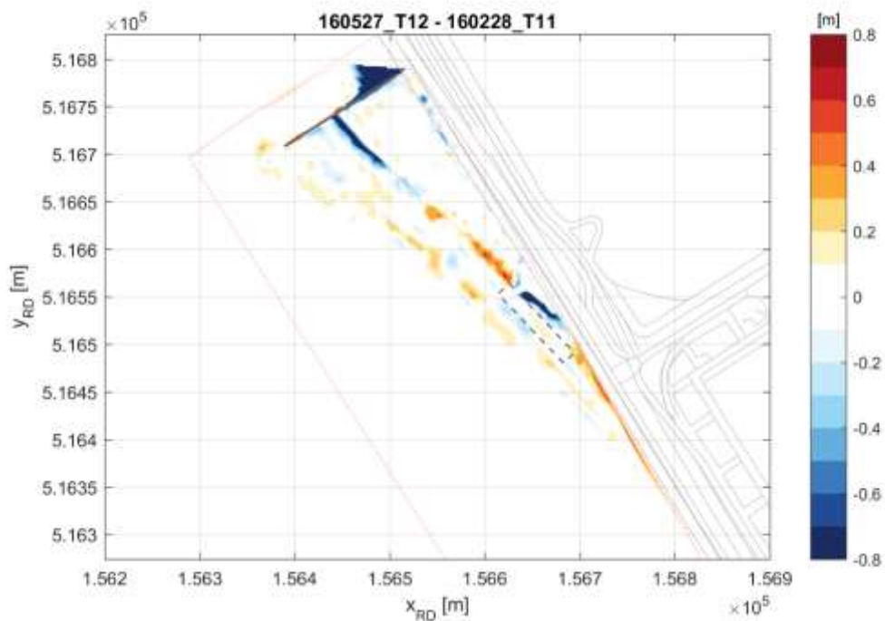
Figuur 6-33 Verschil in bodemligging tussen T11- en T12-opname.
