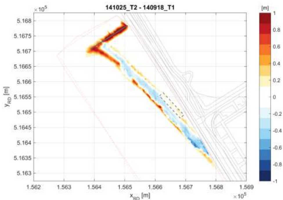
Figuur 6-23 Verschil in bodemligging tussen T1- en T2-opname.
