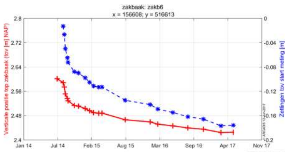
Figuur 6-46 Absolute ontwikkeling top van het zakbaken voor zakb6 (rode lijn), samen met de bijbehorende zetting (blauwe lijn).
