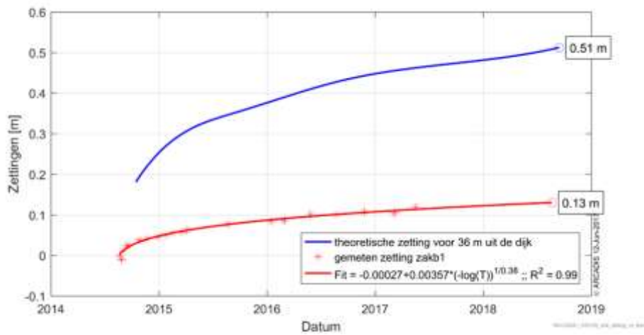
Figuur 6-58 Gemeten zettingen in zakb1 vergeleken met de theoretische zetting voor dit punt.
